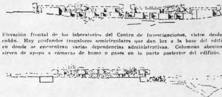
Corte por uno de los jardines de los laboratorios. En primer plano, detrás de los árboles, se ven los estudios de los investigadores, apoyados en columnas sobre el jardín. A la derecha, en corte, pueden verse las dependencias administrativas que forman la base y que dominan el cañón. En el extremo izquierdo, en corte, cuartos subterráneos para animales que son utilizados por los cuatro edificios.
