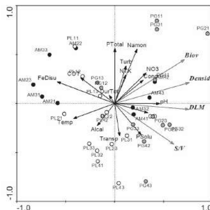
Figura 1. RDA biplot entre épocas. Las estaciones están nombradas según el embalse: AM: Embalse Abreo – Malpaso; PG: Embalse Peñol – Guatapé; PL: Embalse Playas. El primer número hace referencia a la campaña de muestreo, mientras que, el segundo, a la estación.
