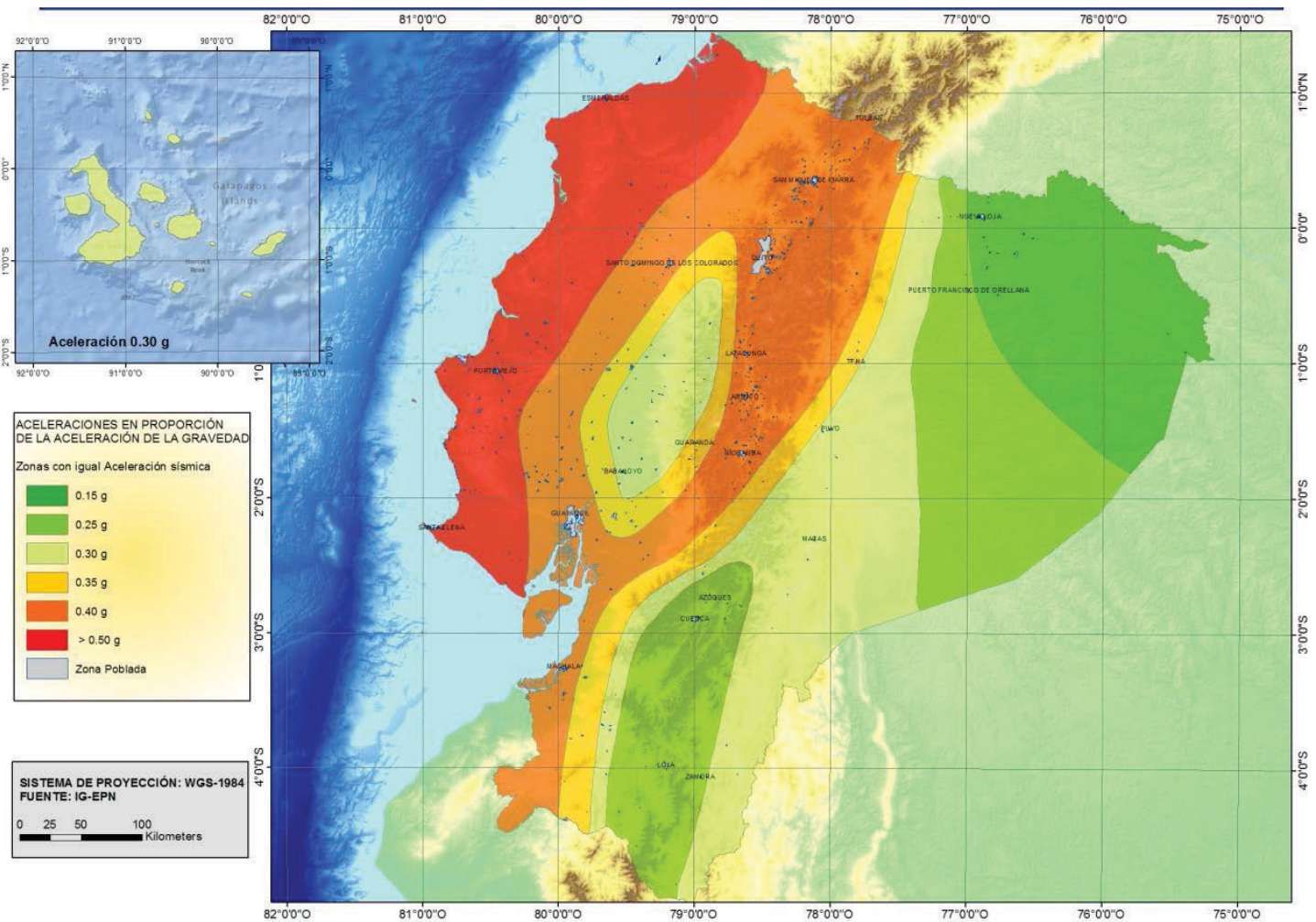
Figura 9. Ecuador, zonas sísmicas para propósitos de diseño y valor del factor de zona Z
