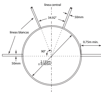
Figura 187c.- Disposición de un Círculo de Martillo
