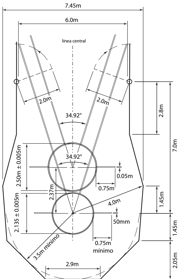
Figura 192c.- Jaula para el Lanzamiento de martillo y Disco con círculos independientes
