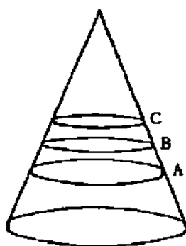
FIG. 9.—La paradoja de Demócrito de las secciones paralelas adyacentes de un cono.
