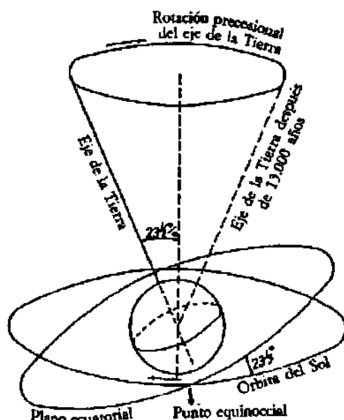
FIG. 2.—Precesión de los equinoccios.
