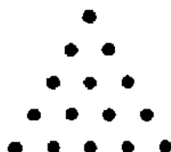
FIG. 1.— Diagramas triangulares.
