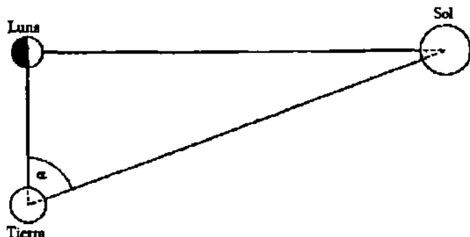
FIG. 6.—La determinación de las distancias relativas Tierra-Sol y Tierra-Luna de Aristarco.
