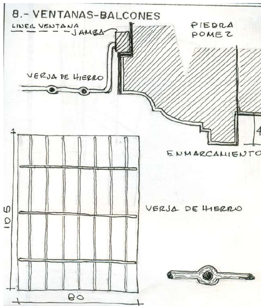
Detalles de ventanas y balcones.
