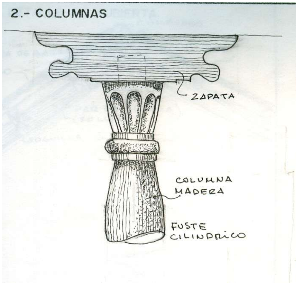
Detalle de columnas.
