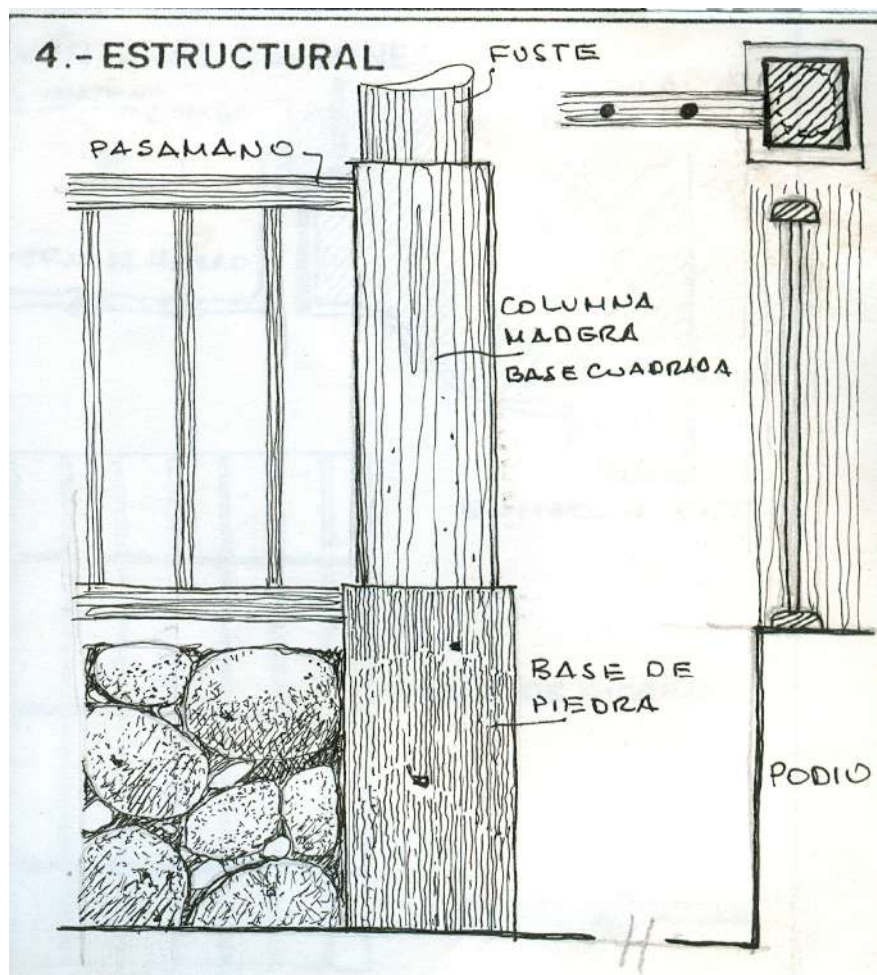
Detalle estructural de soportal.
