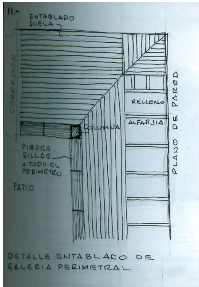
Detalle del entablado de la galería perimetral.
