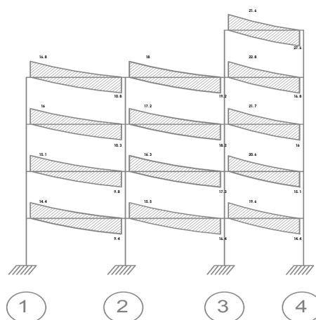
Vu 2cs (T) Pórtico C
