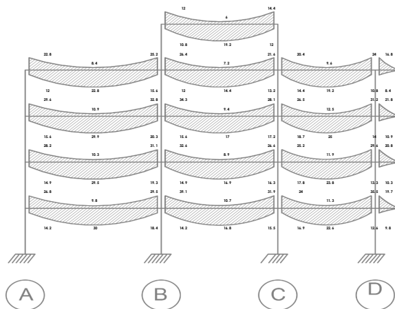
Mu (T-m) Pórtico 3
