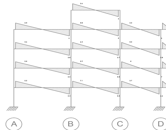
Vu cm(T) Pórtico 3
