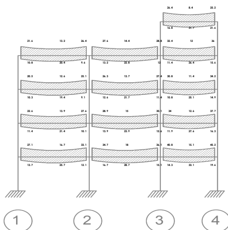
Mu (T-m) Pórtico C
