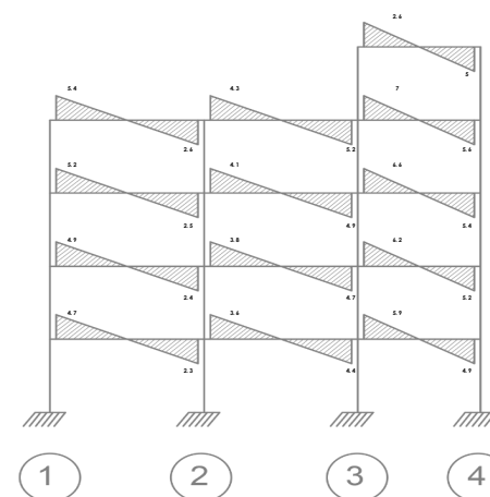
Vu cm(T) Pórtico C
