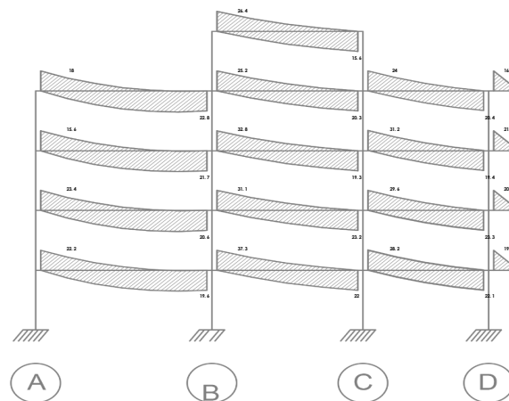
Vu 2cs (T) Pórtico 3
