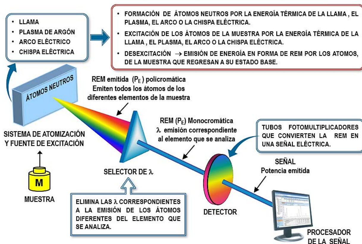
Figura 5.1. Componentes básicos y procesos en un espectrómetro de emisión atómica
