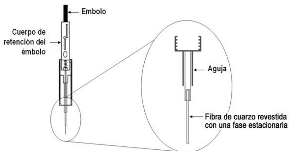
Figura 11.19. Jeringa con la fibra de vidrio recubierta de fase estacionaria
