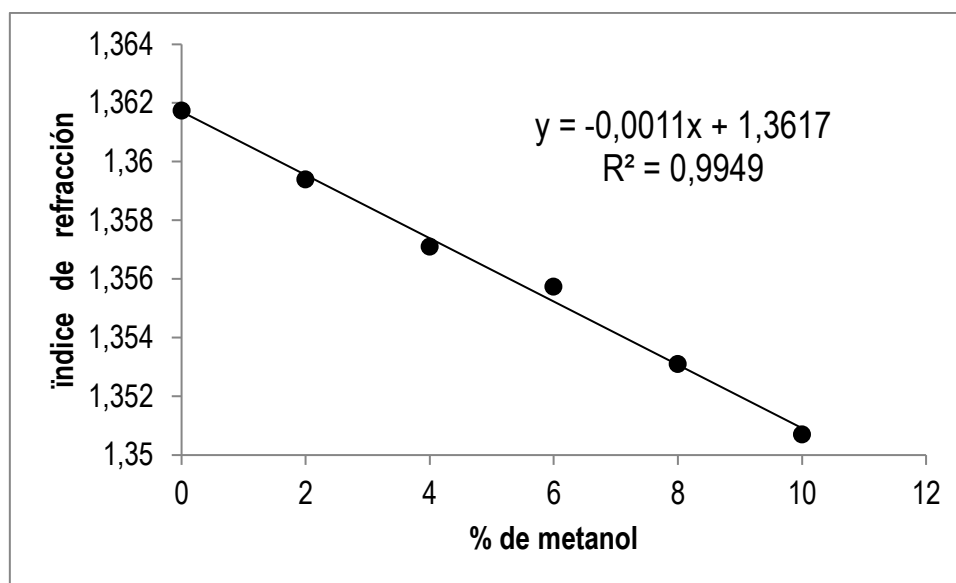
Figura 7.9. Curva de calibración expresada en % de metanol vs. \eta
