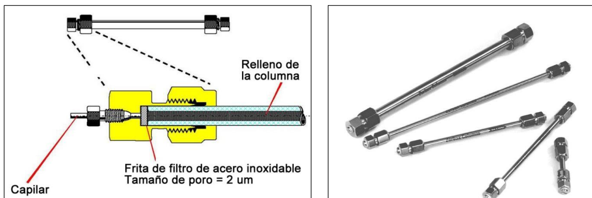
Figura 10.4. Columnas cromatográficas de relleno, de acero inoxidable para HPLC
