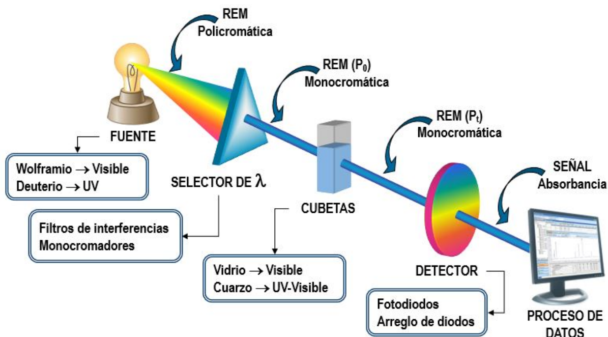
Figura 3.9. Componentes básicos de los instrumentos para medir absorción de radiación.
