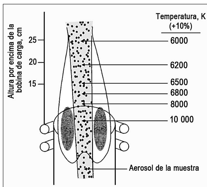
Figura 5.4. Temperaturas en una fuente característica de plasma de acoplamiento inductivo
