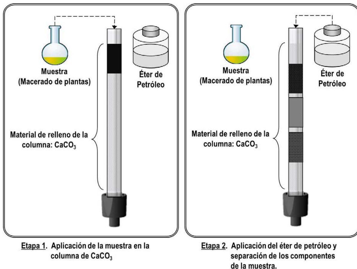
Figura 8.1. Experimento de Mijail Tswett
