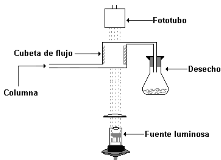
Figura 10.6. Esquema de un detector UV para HPLC
