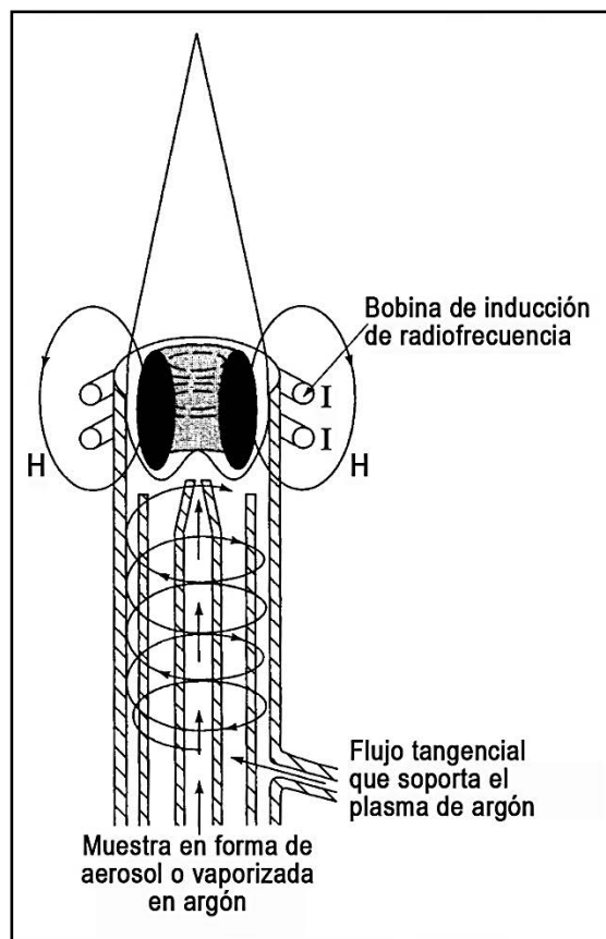
Figura 5.2. Típica fuente de plasma de acoplamiento inductivo
