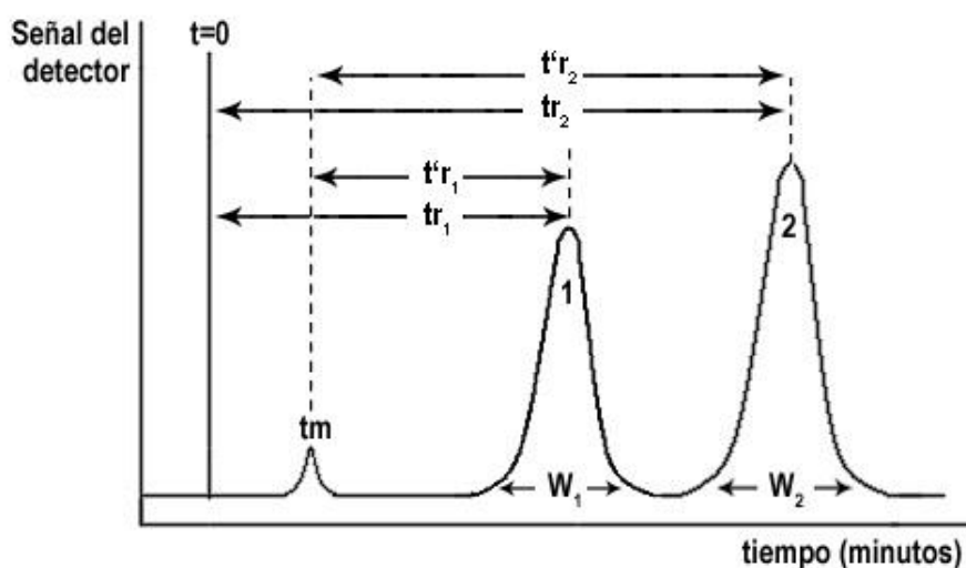
Figura 9.9. Parámetros para el cálculo de la Resolución entre dos picos cromatográficos.
