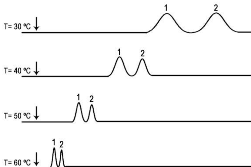
Figura 11.7. Efecto de la temperatura sobre la separación cromatográfica. Nótese que al aumentar la temperatura disminuyen los tiempos de retención ( t_r ) de los compuestos separados, así como también el ensanchamiento de banda. En el ejemplo considerado es beneficioso incrementar la temperatura por cuanto se pretende disminuir los t_r , sin embargo, en el caso que se obtengan cromatogramas con picos solapados a bajos tiempos de retención, convendría disminuir la temperatura para mejorar la resolución.
