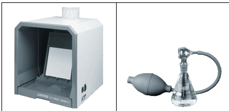
Figura 12.16. Cámara de pulverización y pulverizador para atomización
