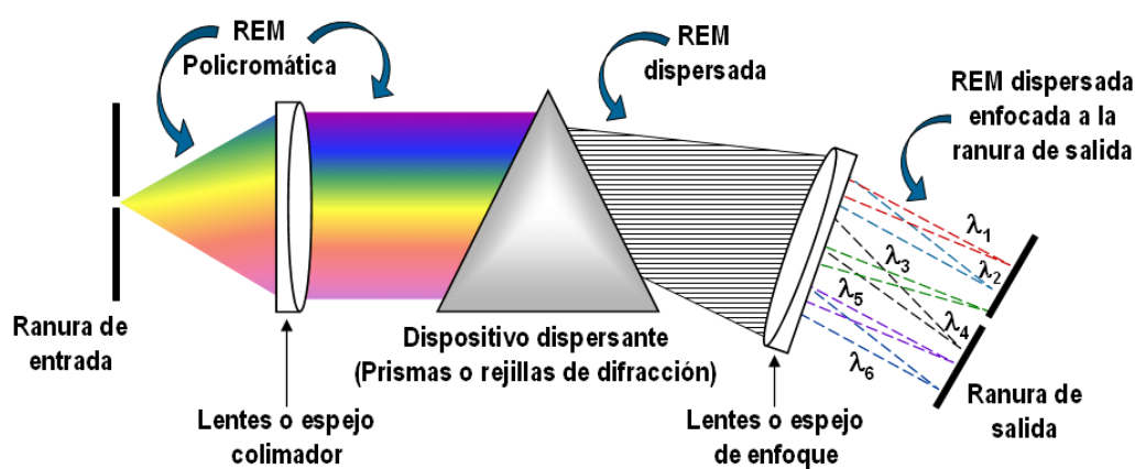
Figura 3.10. Esquema general de un monocromador. La radiación penetra por una ranura de entrada, es colimada por un lente que produce haces de radiación paralela, los cuales llegan al dispositivo dispersante y son dispersados por refracción (prismas) o difracción (rejillas). Los haces de radiación monocromática son enfocados luego enfocados hacia la ranura de salida. Haciendo girar el dispositivo dispersante, se logra que la radiación de la longitud de onda deseada atraviese la ranura de salida.
