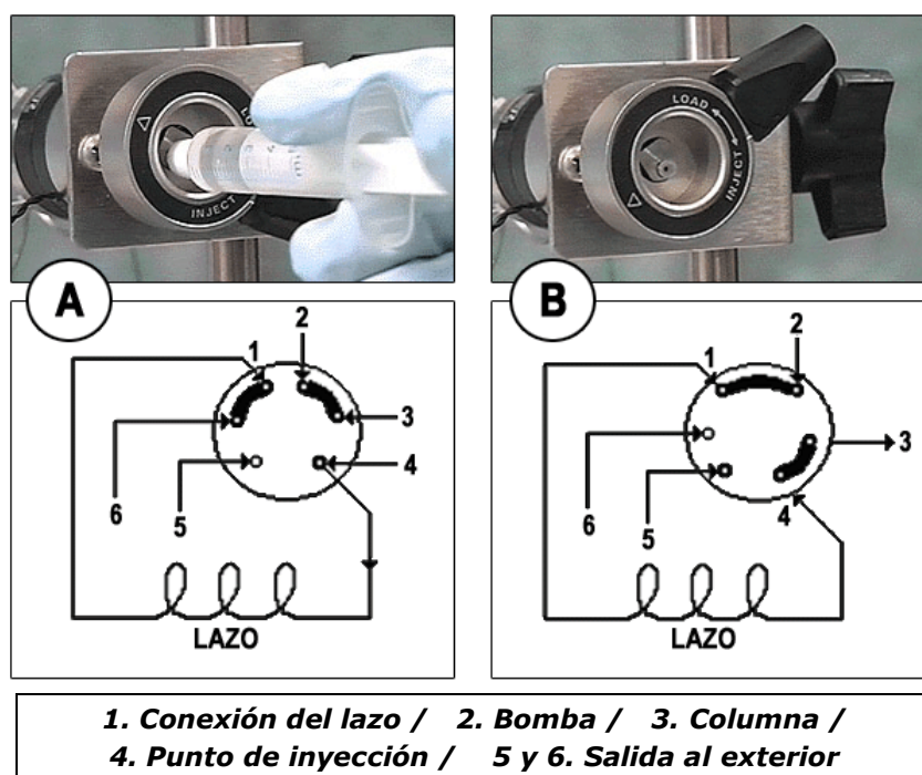
Figura 10.2. Válvula de inyección: A) posición de carga, B) introducción a la columna
