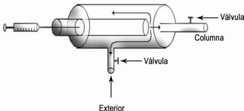
Figura 11.3. Esquema simplificado de un inyector Split
