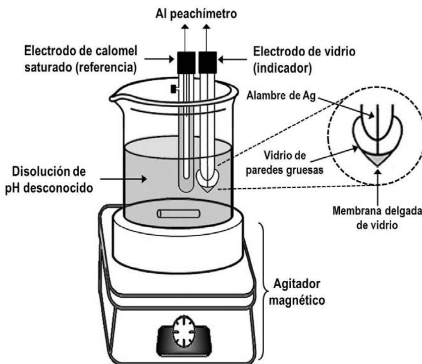
Figura 13.4. Sistema de electrodos típico para medir pH
