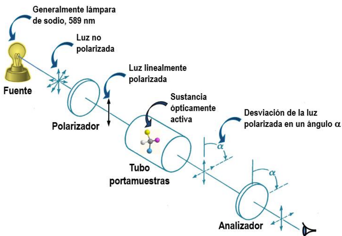
Figura 7.11. Esquema general de un polarímetro
