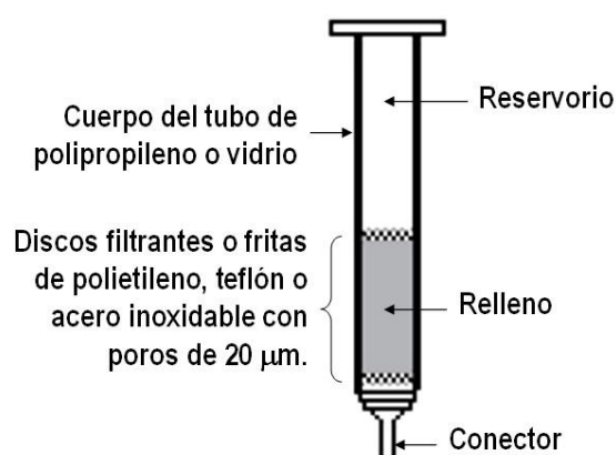
Figura 10.15. Cartucho de extracción en fase sólida
