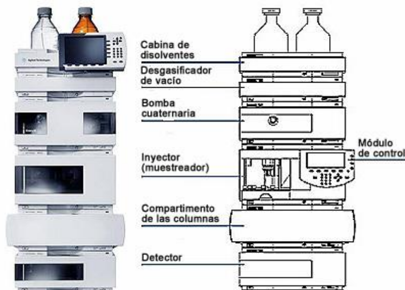
Figura 10.9. Diseño modular de un cromatógrafo líquido de alta resolución (HPLC) de la serie 1200, comercializado por la firma alemana Agilent Technologies
