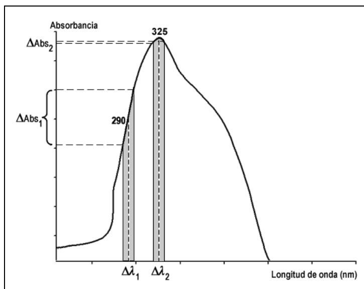
Figura 3.12. Influencia de la variación de la longitud de onda sobre la medición de absorbancia.
