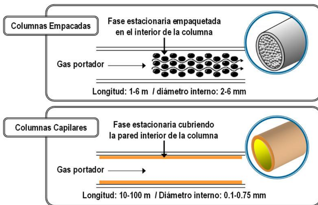
Figura 11.4. Columnas para cromatografía de gases
