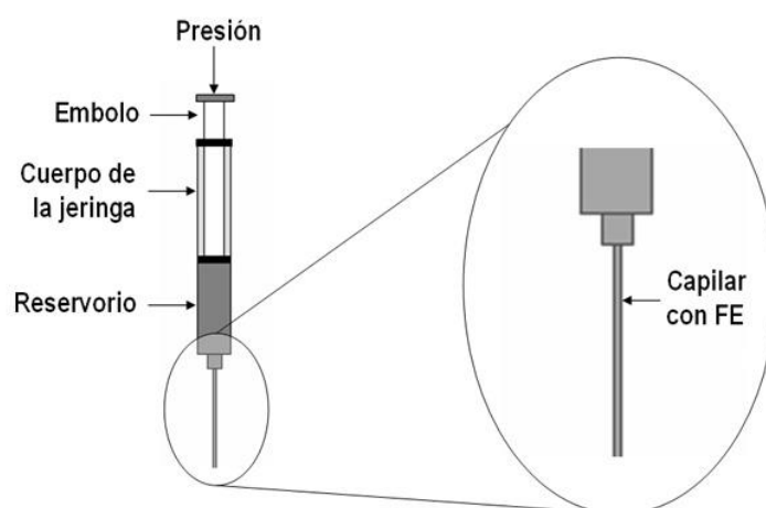
Figura 10.16. Jeringa con el capilar contentivo de la fase estacionaria
