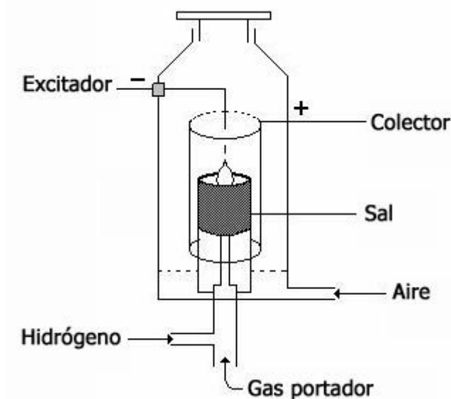
Figura 11.16. Detector termiónico
