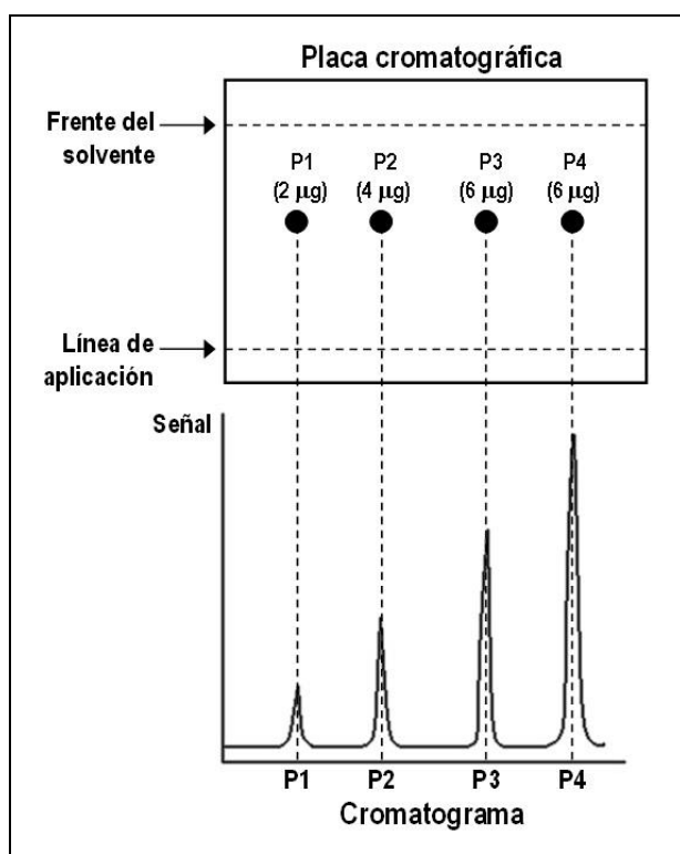
Figura 12.19. Curva de calibración y detección densitométrica.
