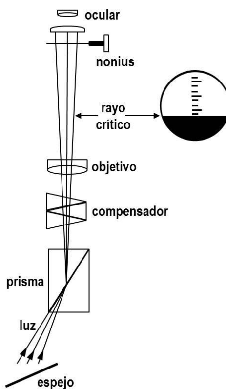
Figura 7.6. Esquema de un refractómetro de inmersión.
