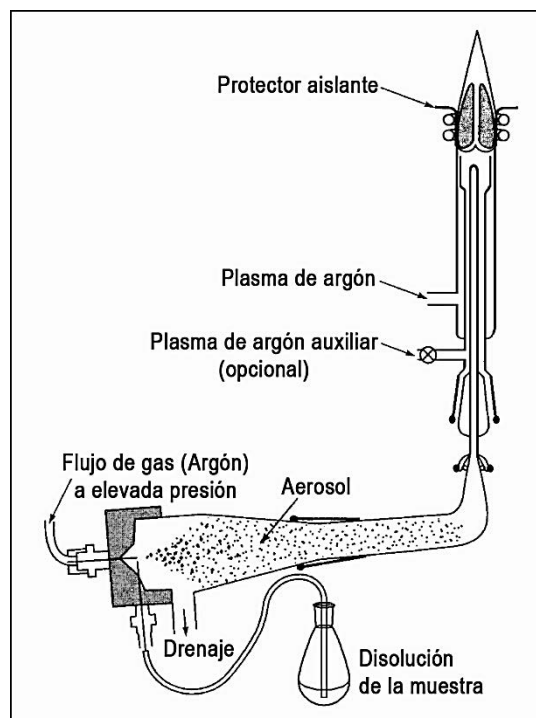
Figura 5.3. Típico nebulizador neumático para la inyección de la muestra en una fuente de plasma.
