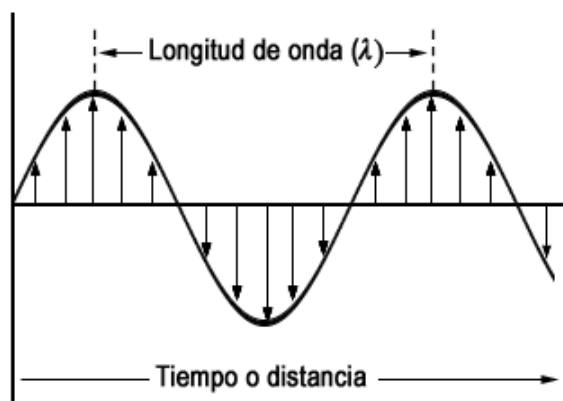
Figura 2.1. Representación de un haz de radiación monocromática polarizada en un plano. Las flechas representan el vector eléctrico.
