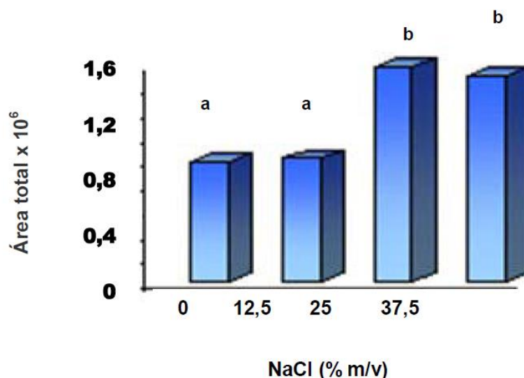
Figura 2. Influencia de la concentración salina en el área total de los picos. Fibra CAR/PDMS, 8 mL de cerveza, 15 min de pre-extracción y 2 min de desorción. Letras distintas indican diferencias significativas para p \leq 0,05 .
