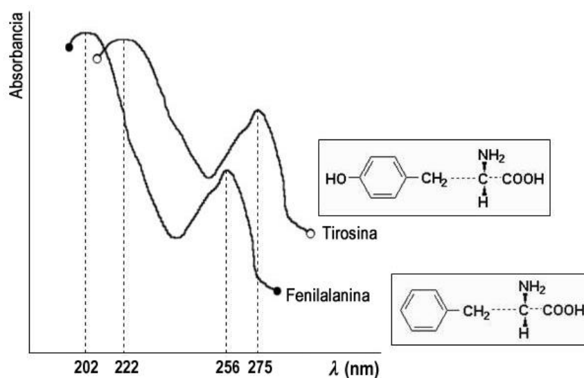
Figura 3.7. Desplazamiento de las longitudes de onda máximas por efecto de la sustitución de un grupo OH. Nótese que las estructuras de la Tirosina y la Fenilalanina son casi idénticas. El grupo OH de la Tirosina provoca un efecto batocrómico del espectro hacia valores mayores de longitudes de onda con respecto a la Fenilalanina.
