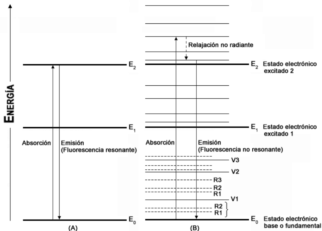
Figura 2.7. Procesos de emisión. (A). Fluorescencia resonante, característica de los procesos de emisión atómica, en la que se emite una radiación de igual frecuencia que la absorbida. (B). Fluorescencia no resonante, característica de los procesos de emisión molecular, en la que generalmente se emite una radiación de menor frecuencia (mayor longitud de onda) que la absorbida, debido a fenómenos de relajación vibratoria.
