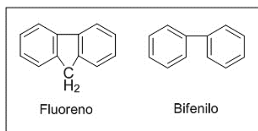
Figura 6.3. Efecto de la rigidez estructural en la fluorescencia
