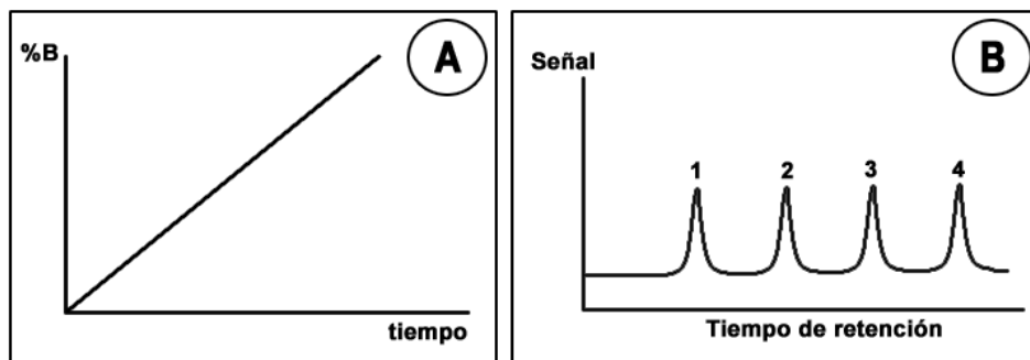
Figura 10.12. Gradiente lineal: (A) representación gráfica, (B) cromatograma característico.
