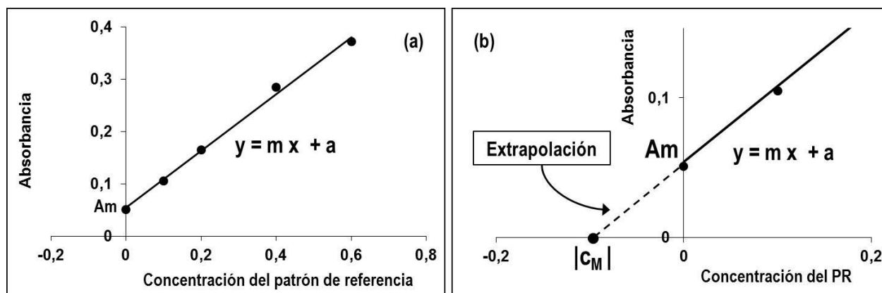
Figura 4.10. (a) Comportamiento gráfico de una curva de adición de patrón, (b) Extrapolación de la curva hacia la zona negativa del eje x para el cálculo de la concentración de la disolución de muestra problema c_M .
