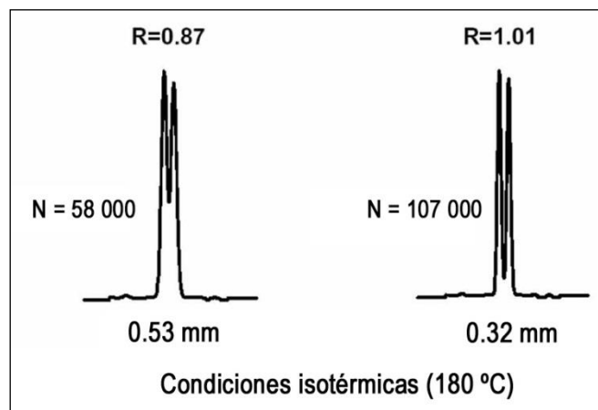
Figura 11.6. Efecto del diámetro interno de la columna sobre la resolución.
