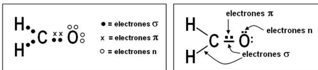
Figura 3.5. Dos maneras de representar los diferentes tipos de electrones en la molécula de formaldehído
