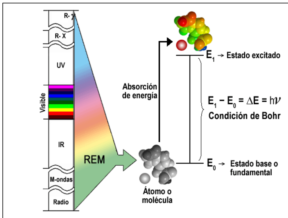
Figura 2.3. Representación esquemática del proceso de absorción de radiación.
