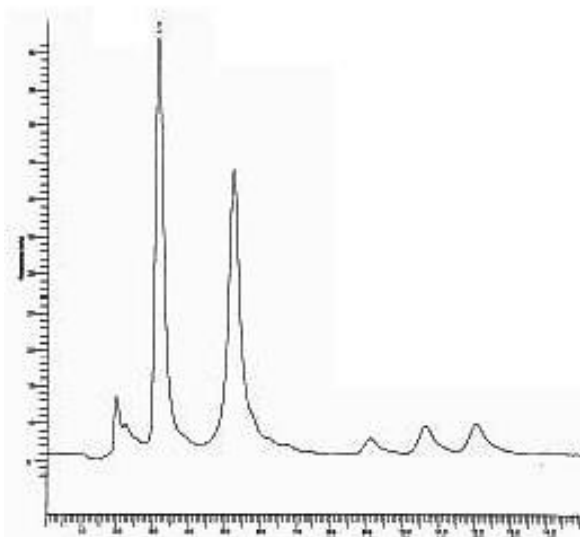
Figura 1. Perfil cromatográfico de las derivatizaciones de Aflatoxina M_1 y B_1 con ácido trifluoroacético.
