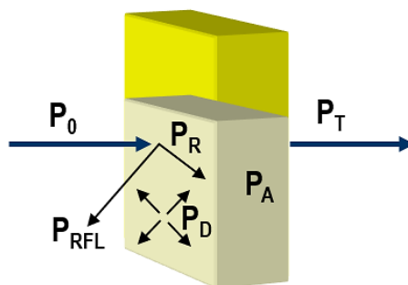
Figura 3.3. Fenómenos que ocurren cuando un haz de radiación electromagnética incide sobre una solución de sustancia contenida en un recipiente ( P_0 = Potencia incidente, P_{RFL} = Potencia reflejada, P_{RFR} = Potencia refractada, P_D = Potencia dispersada, P_A = Potencia Absorbida, P_T = Potencia transmitida).
