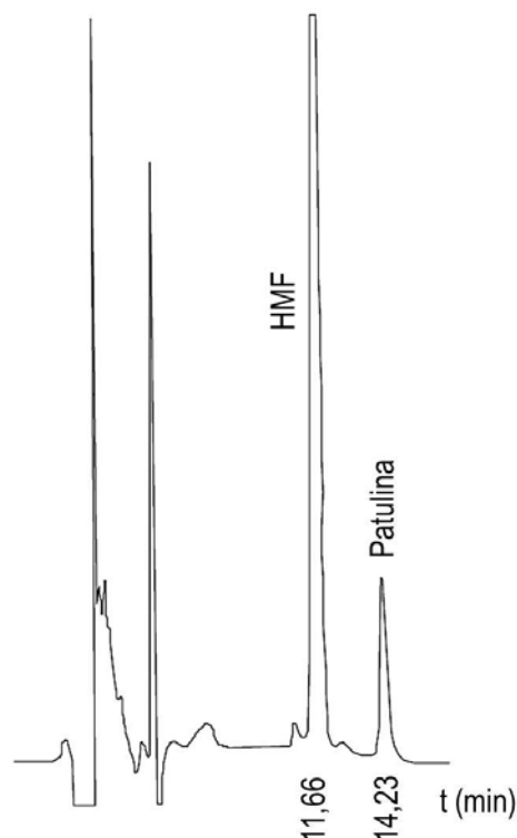
Figura 3. Cromatograma de una muestra de jugo de manzana contaminada con 3 µg/L.
