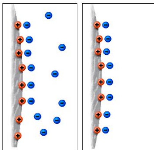
Figura 8.6. Equilibrio de la resina
