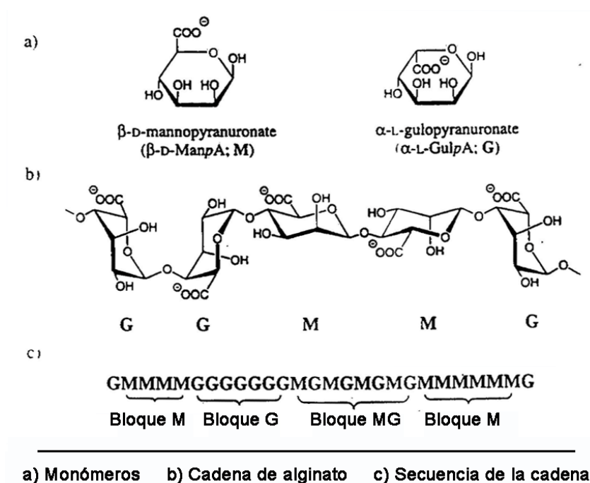
Figura 1. Estructura del ácido algínico
