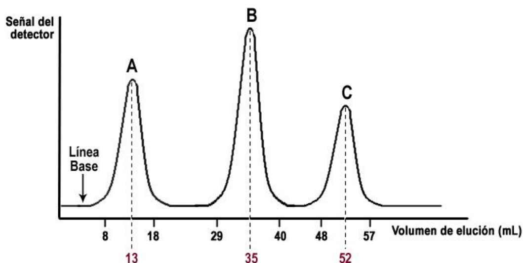
Figura 9.5. Cromatograma de señal vs. volumen de elución
