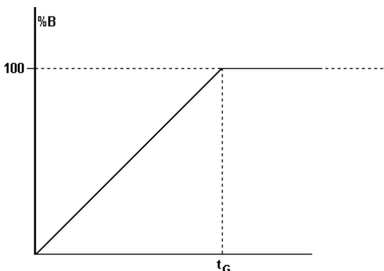
Figura 10.11. Incremento lineal del solvente B. Tiempo de gradiente ( t_G )
