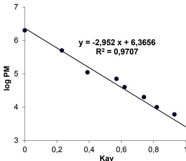
Figura 3. Calibración de columna en la determinación del peso molecular
