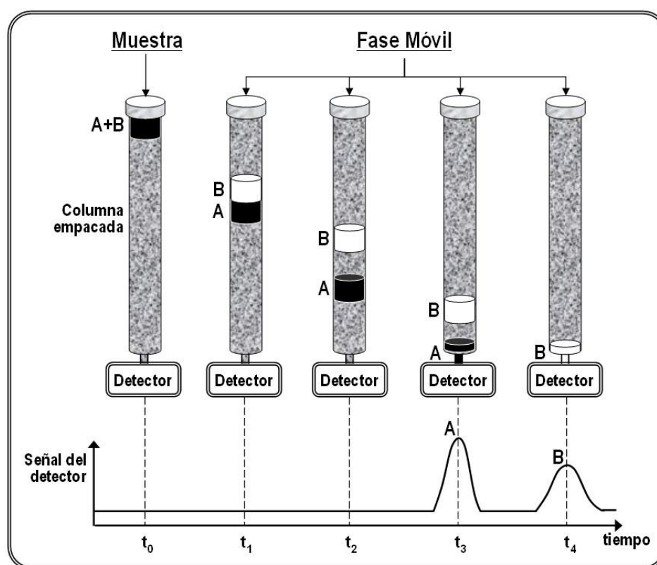
Figura 9.1. Etapas de la separación cromatográfica
