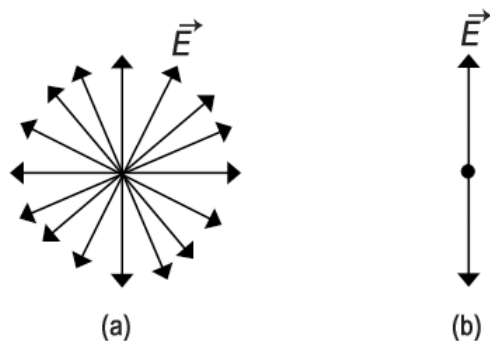
Figura 2.9. (a) Una onda transversal no polarizada que se mueve hacia el lector, vista como una superposición al azar de muchos trenes de ondas polarizados, (b) Una onda transversal polarizada en un plano. En ambas figuras se muestra solo el vector eléctrico ( \vec{E} ).
