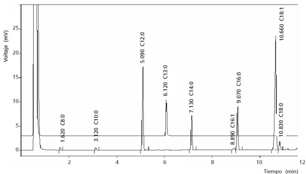
Figura 1. Superposición de los perfiles cromatográficos de D-004 (superior) y ácido tridecanoico (C 13:0 ) utilizado como estándar interno. Todos analizados como ésteres metílicos
