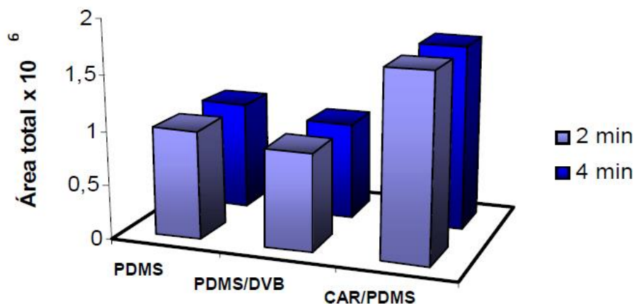
Figura 1. Comparación de las fibras con distintos tiempos de desorción
