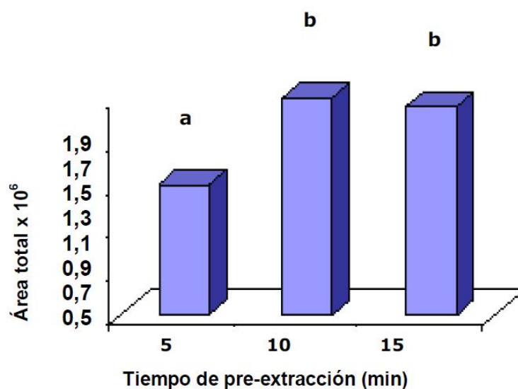
Figura 3. Influencia del tiempo de pre-extracción en el área total. Fibra CAR/PDMS, 8 mL de cerveza, 2 g de NaCl y 2 min de desorción. Letras distintas indican diferencias significativas para p \leq 0,05 .
