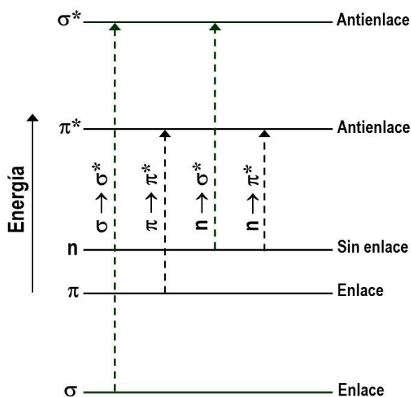
Figura 3.6. Niveles electrónicos de energía molecular.
