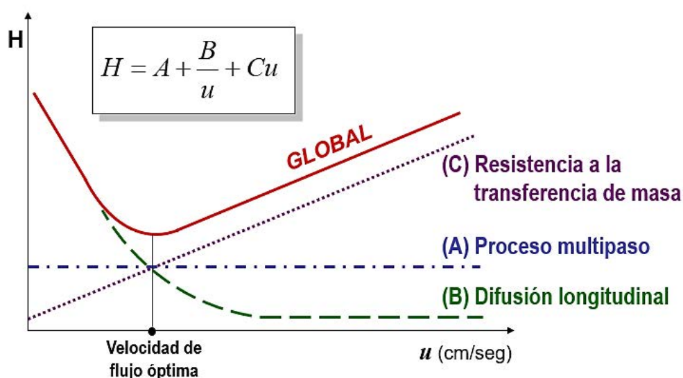
Figura 9.14. Solución gráfica de la ecuación de Van Deemter.
