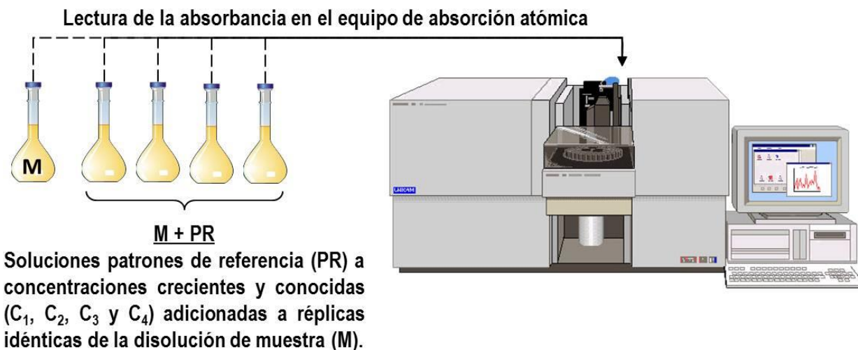
Figura 4.9. Procedimiento de preparación y lectura de una curva de adición de patrón.
