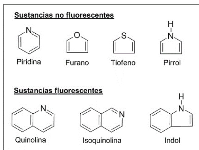
Figura 6.2. Efecto de la condensación estructural en la fluorescencia
