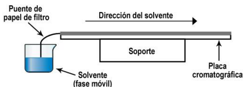
Figura 12.10. Desarrollo horizontal convencional
