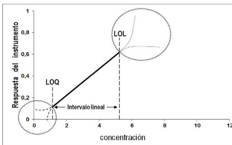
Figura 1.3. Intervalo lineal de un método analítico. LOQ= límite de cuantificación, LOL= límite de linealidad
