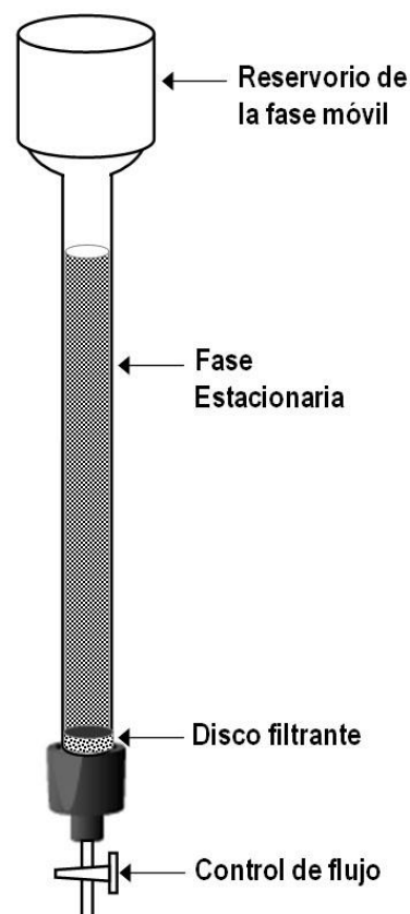
Figura 9.2. Columna cromatográfica con reservorio de solvente
