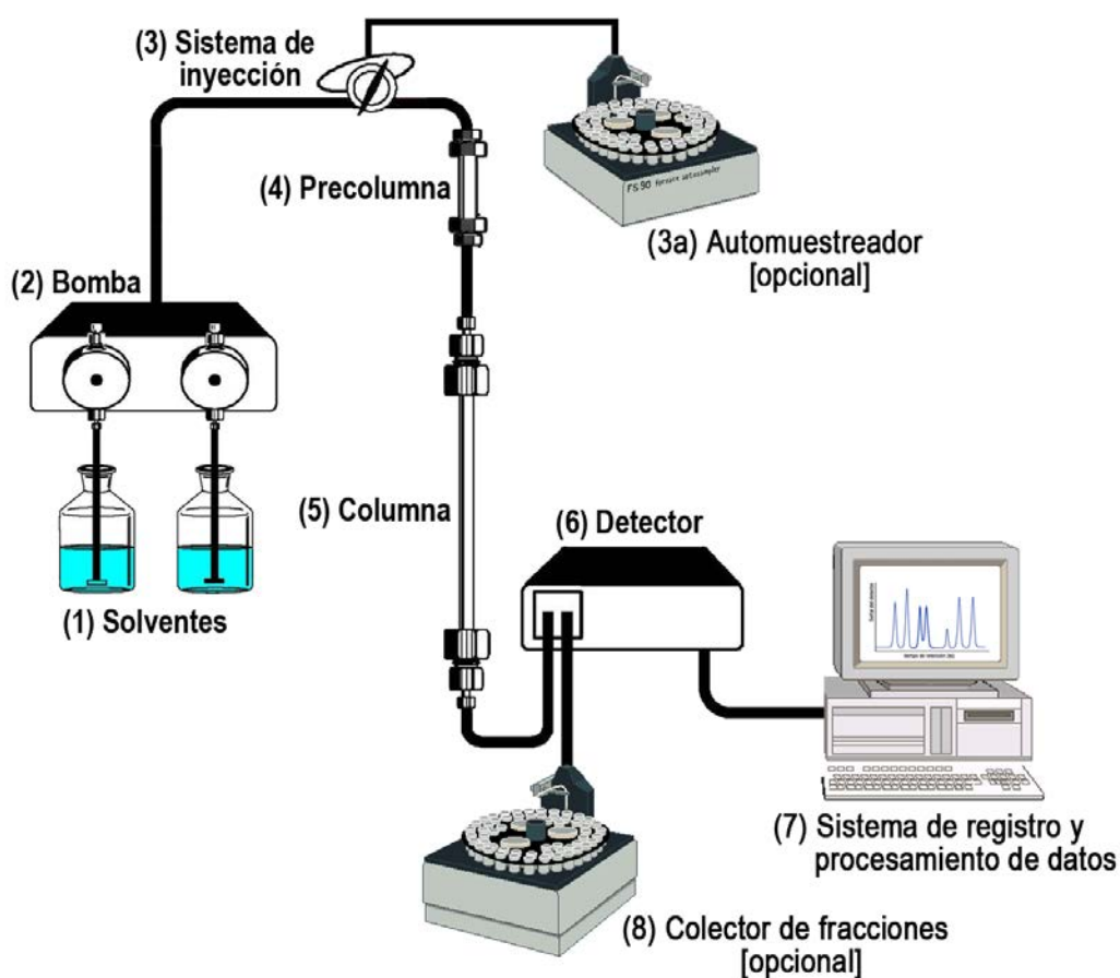
Figura 10.1. Esquema de un sistema cromatográfico HPLC
