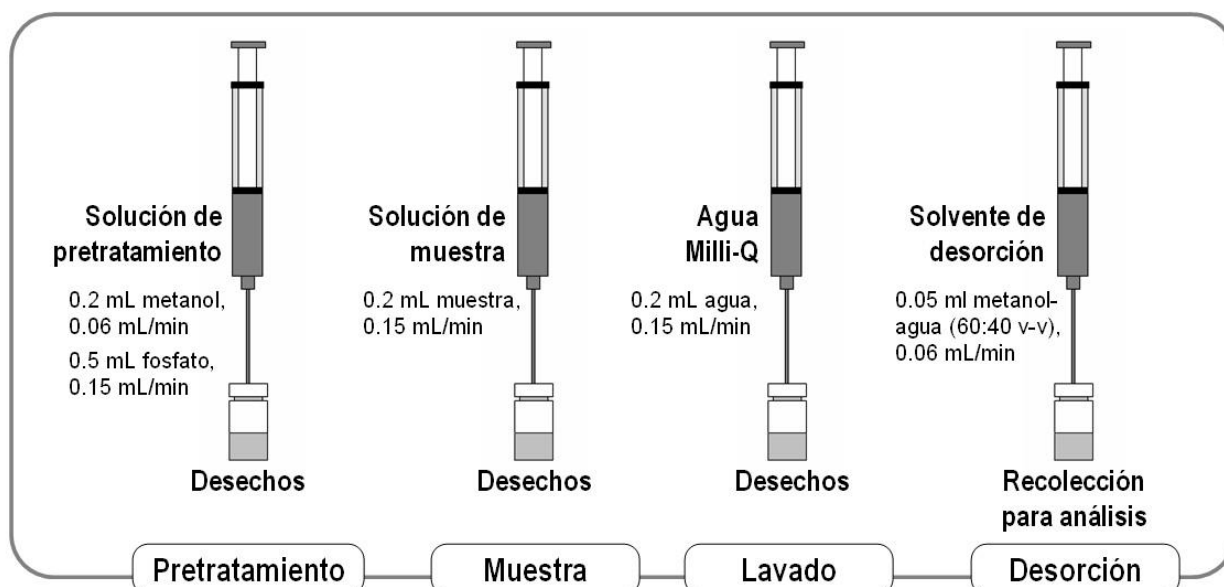
Figura 10.17. Extracción de cloranfenicol el mieles, leche y huevos utilizando microextracción con polímeros monolíticos (ácido metacrílico-dimetilcrilato de etilenglicol)
