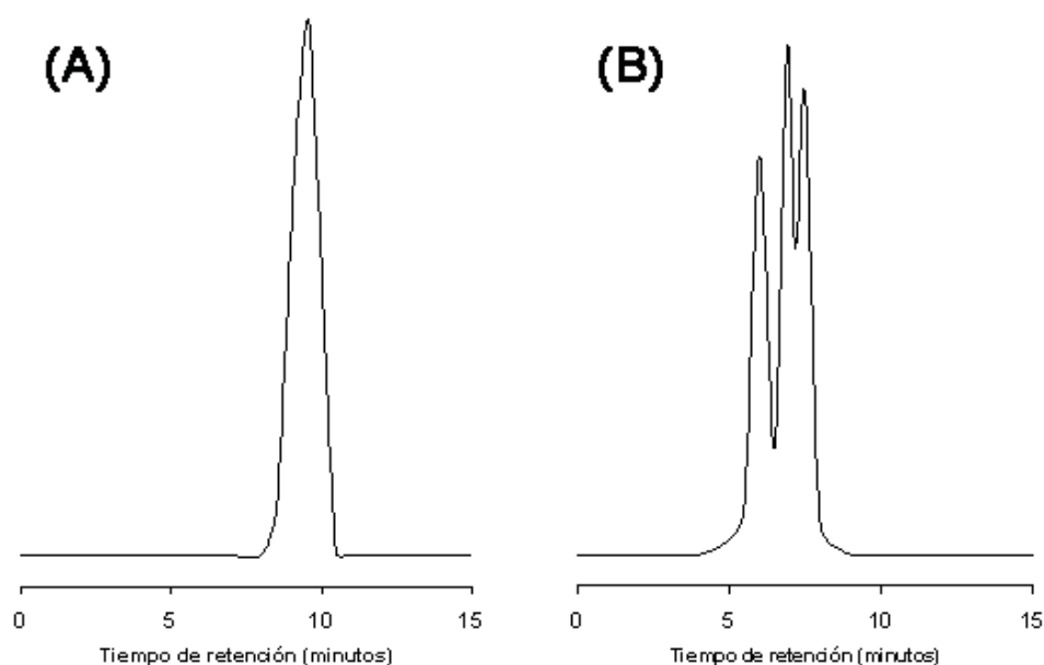
Figura 4. Cromatogramas obtenidos en la determinación del peso molecular para el alginato cubano (A) y el alginato mexicano (B).
