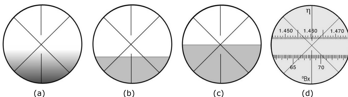
Figura 7.4. Procedimiento de lectura del índice de refracción de una muestra
