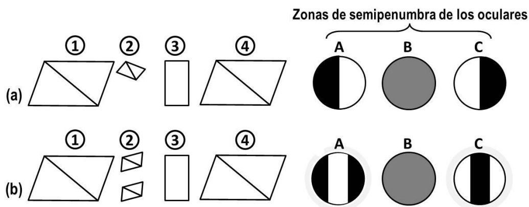
Figura 7.12. Representación esquemática de los sistemas de semipenumbra. (a) con un prisma de Lippich, (b) con dos prismas de Lippich. ① Polarizador, ② Prismas de Lippich, ③ Tubo de muestras, ④ Analizador.
