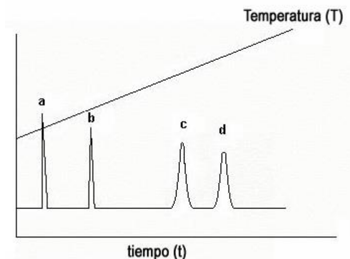
Figura 11.10. Programación lineal de temperatura.
