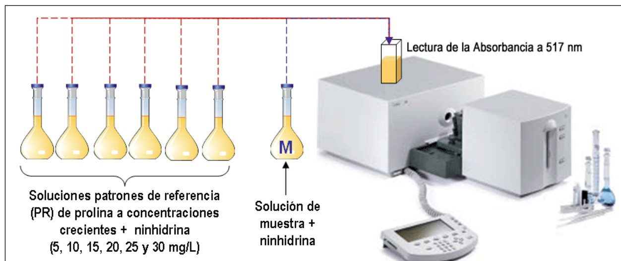
Figura 3.13a. Representación esquemática del procedimiento de curva de calibración para la determinación de prolina en jugo de uvas.
