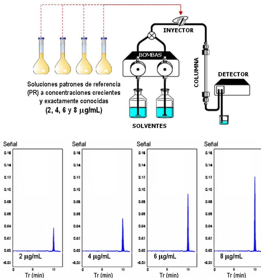
Figura 10.19. Esquema del procedimiento de curva de calibración
