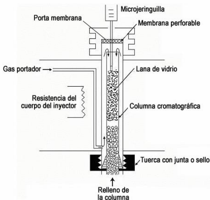
Figura 11.2. Cámara de inyección clásica
