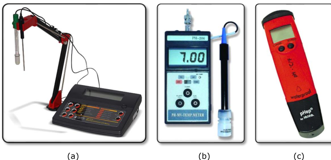
Figura 13.6. Peachímetros comerciales, (a) de mesa, (b) y (c) manuales.
