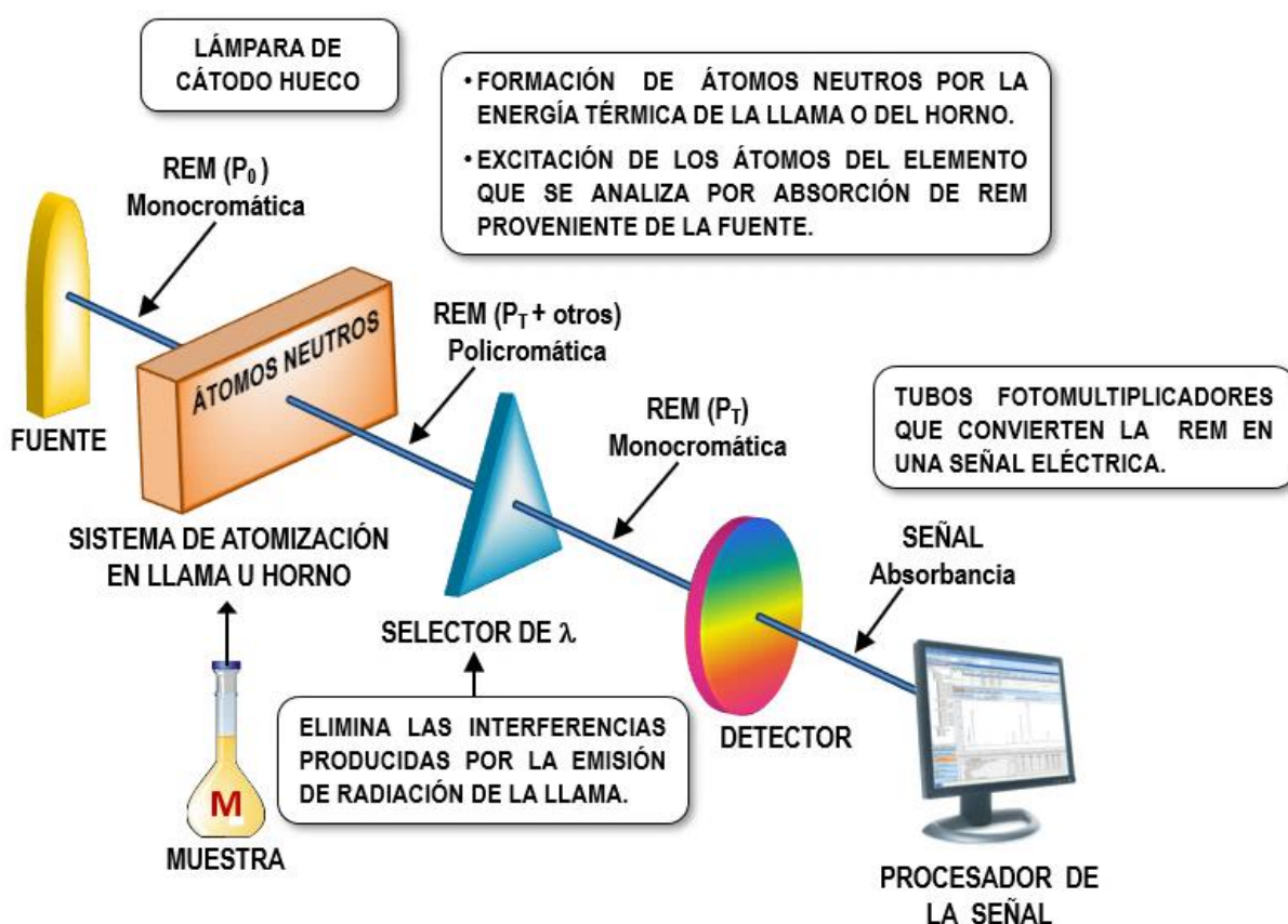
Figura 4.2. Componentes básicos y procesos en un espectrómetro de absorción atómica.
