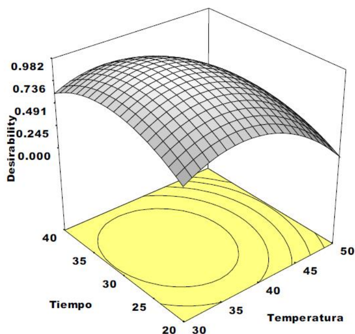
Figura 4. Superficie de respuesta para la optimización del tiempo y temperatura de extracción
