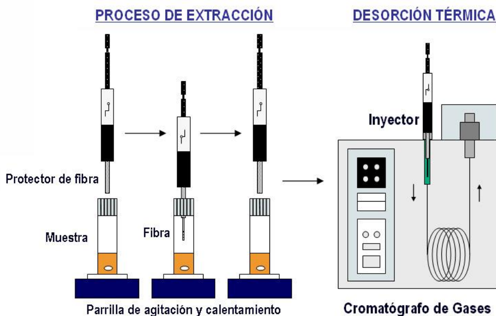
Figura 11.20. Proceso de extracción de volátiles mediante HS-SPME y posterior desorción térmica
