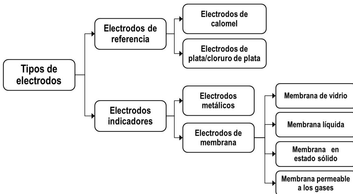
Figura 13.2. Tipos de electrodos usados en los métodos potenciométricos.
