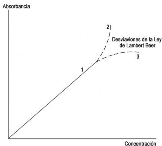
Figura 3.4. Cumplimiento y desviaciones de la ley de Lambert-Beer. (1) cumplimiento de la ley, (2) desviación positiva, (3) desviación negativa
