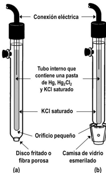
Figura 13.3. Electrodos de referencia de Calomel típicos
