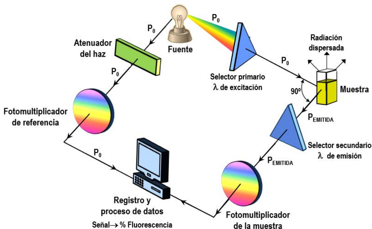
Figura 6.6. Componentes de un fluorómetro o un espectrofluorímetro.
