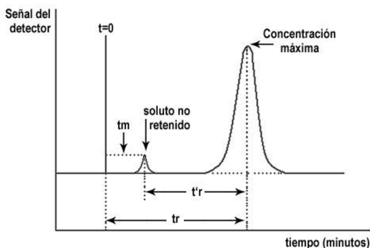
Figura 9.8. Tiempos de retención y otras magnitudes cromatográficas.
