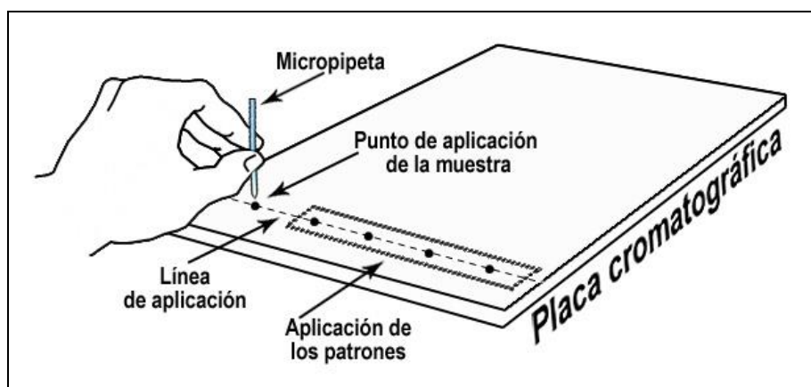
Figura 12.2. Aplicación de la muestra y los patrones
