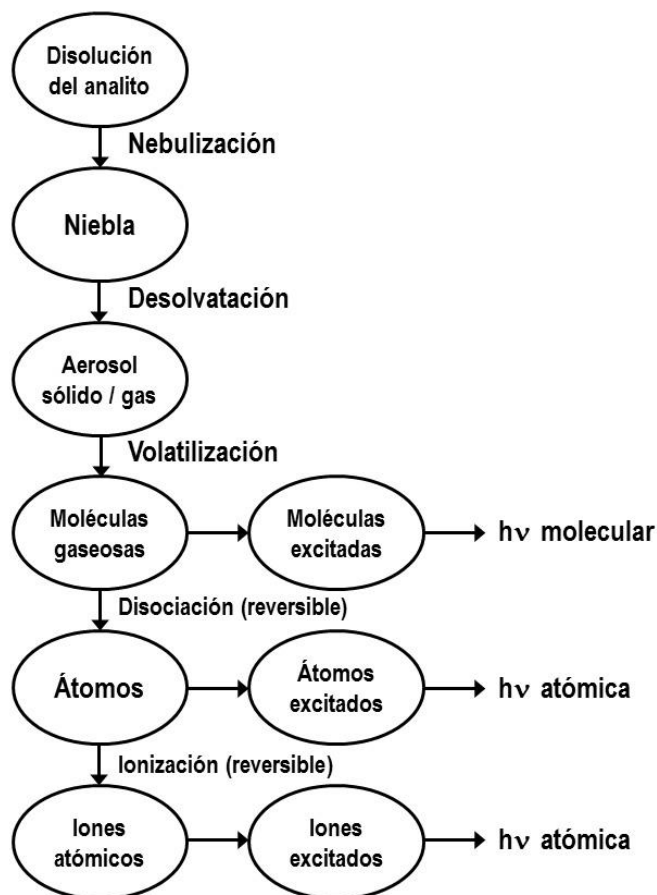
Figura 4.3. Procesos que tienen lugar durante la atomización
