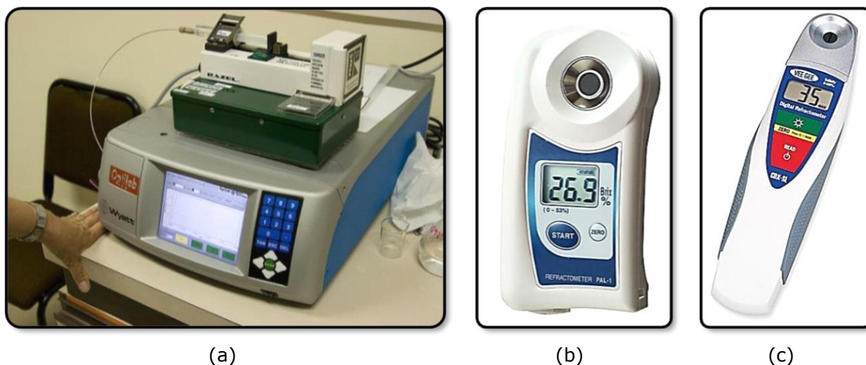
Figura 7.8. Algunos diseños de refractómetros automáticos digitales: (a) de sobremesa; (b) y (c) portátiles.
