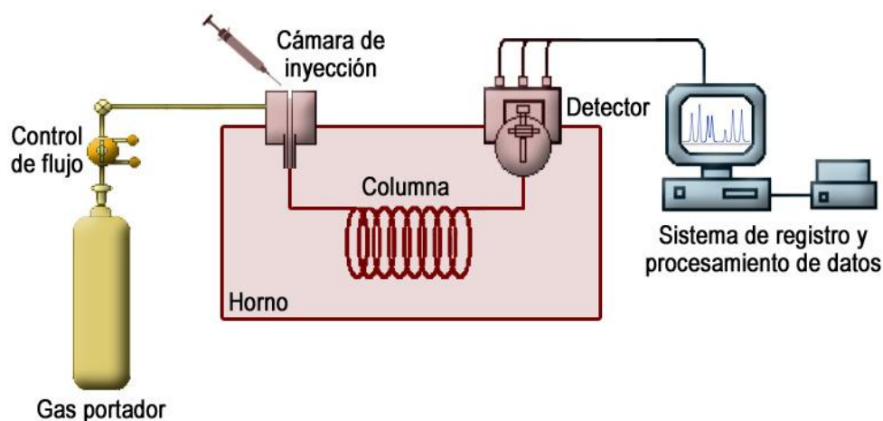
Figura 11.1. Esquema de un sistema de cromatografía de gases
