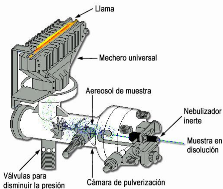
Figura 4.6. Mechero de flujo laminar
