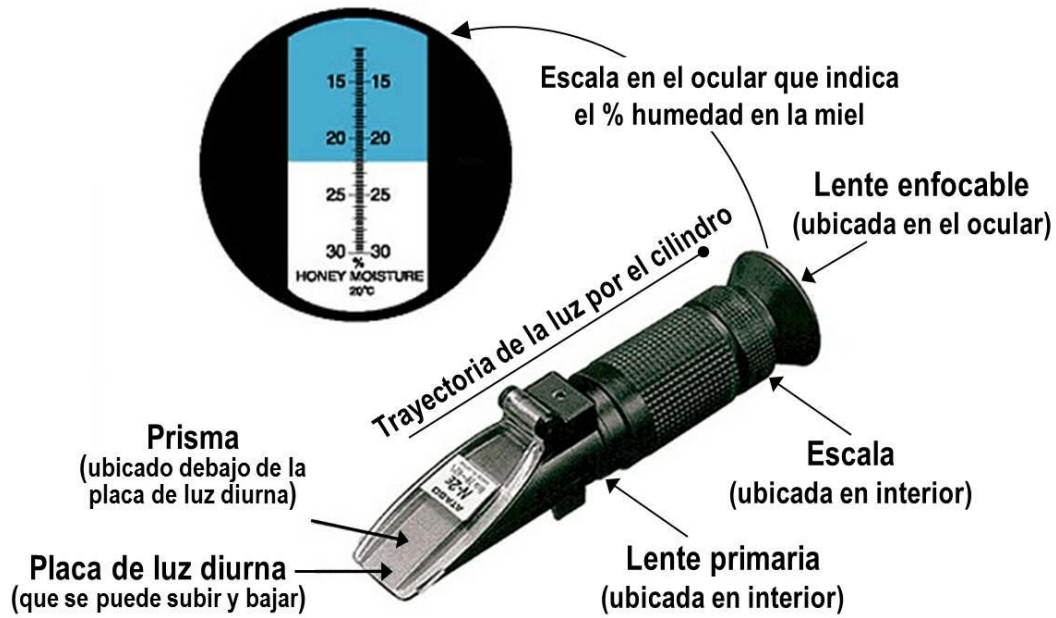
Figura 7.7. Diseño de un refractómetro de inmersión para la medición de humedad en mieles.
