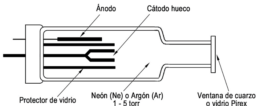
Figura 4.8. Sección transversal de una lámpara de cátodo hueco.
