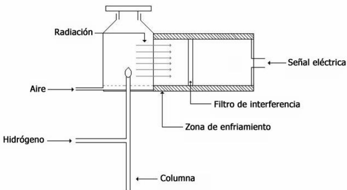
Figura 11.17. Detector fotométrico de llama
