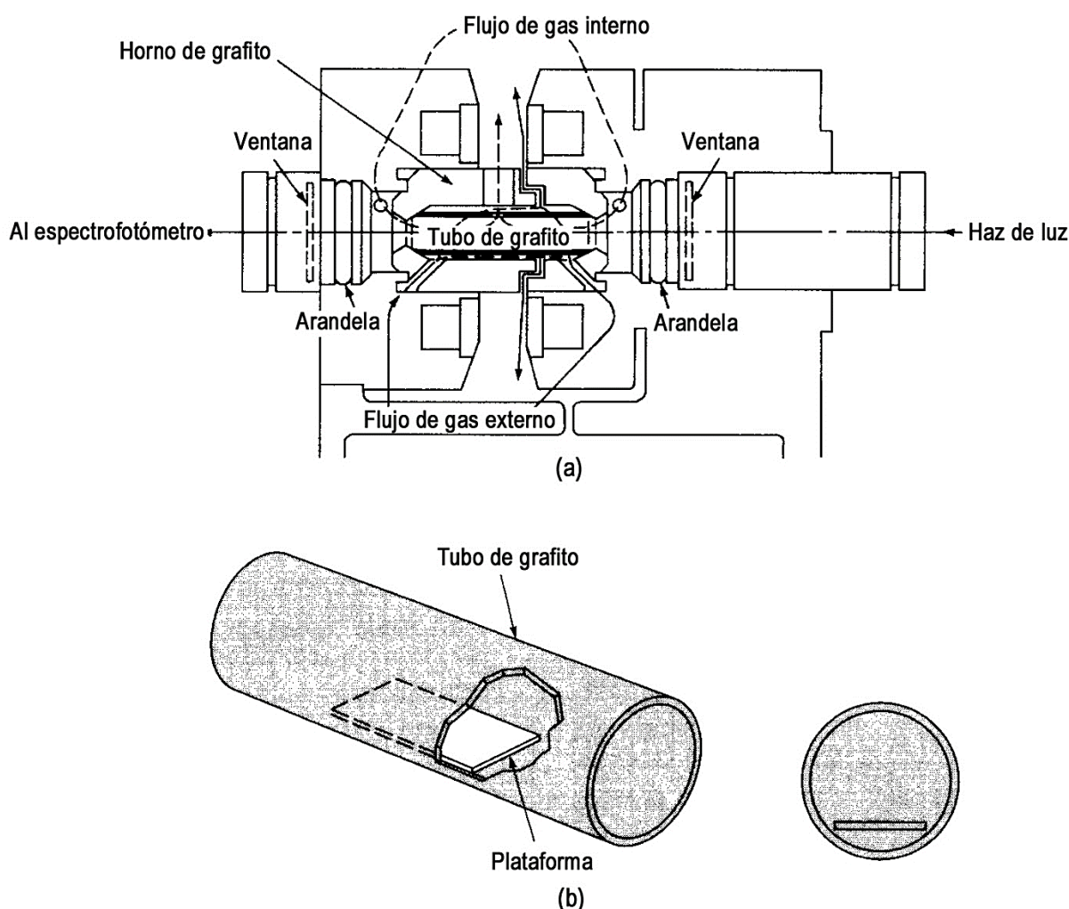
Figura 4.7. (a) Sección transversal de un horno de grafito, (b) Plataforma de L'vov y su posición en el horno de grafito.
