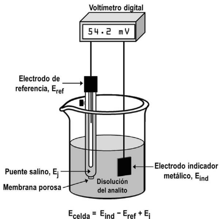
Figura 13.1. Celda para medidas potenciométricas.
