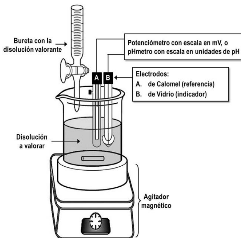
Figura 13.7. Aparato para realizar una valoración potenciométrica
