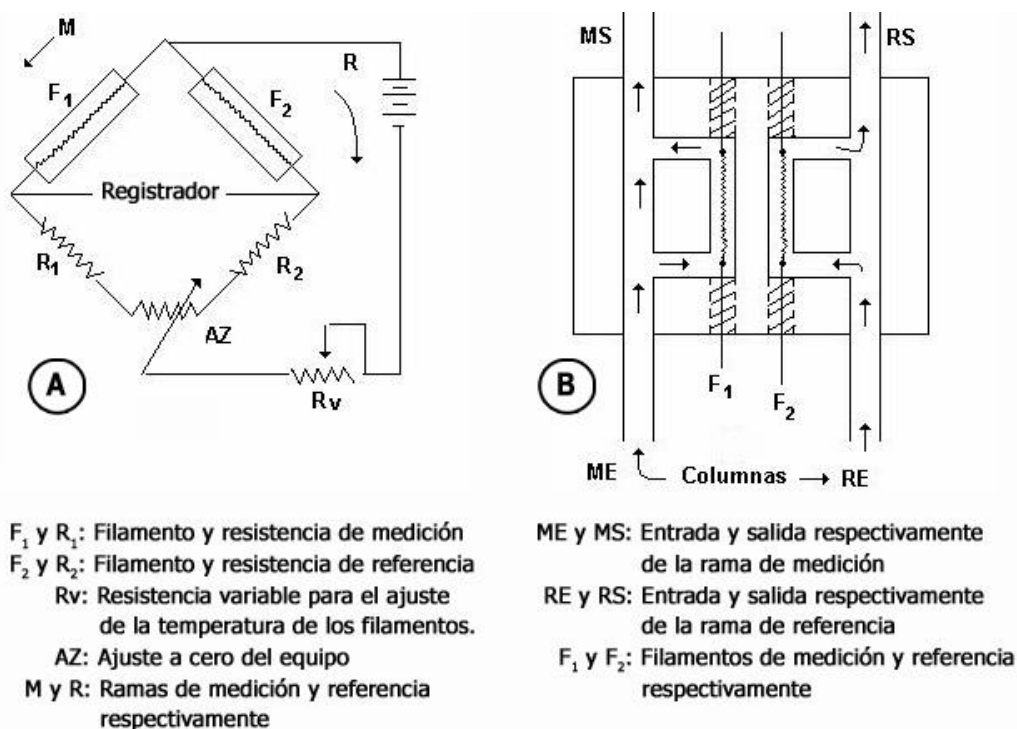
Figura 11.13. Detector de conductividad térmica (TCD)
