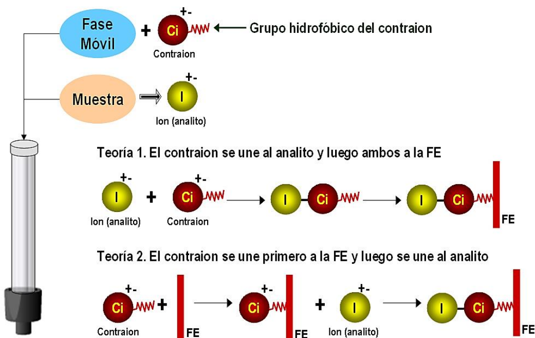
Figura 10.5. Mecanismo de fase reversa – par iónico
