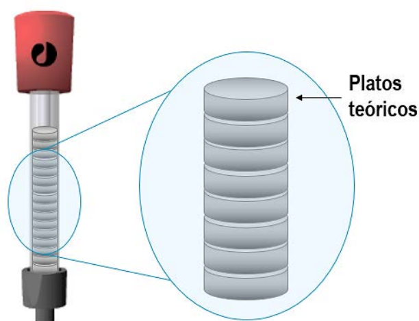
Figura 9.11. Representación esquemática de los platos teóricos
