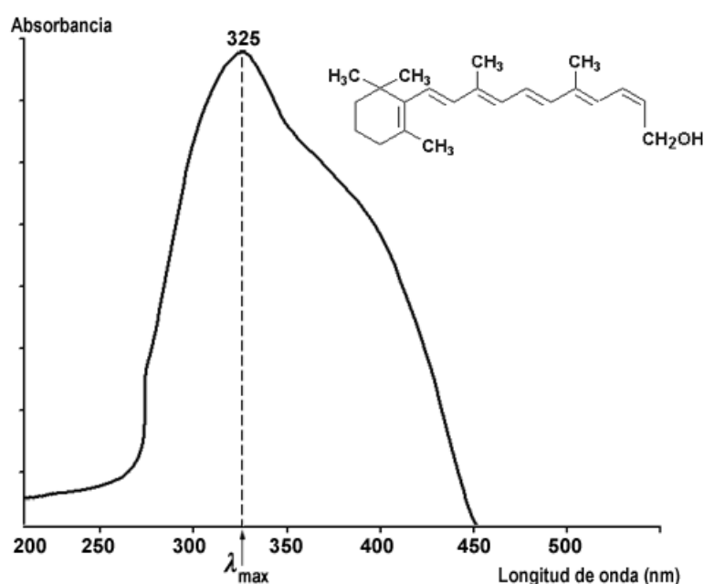
Figura 3.2. Espectro de absorción del Retinol
