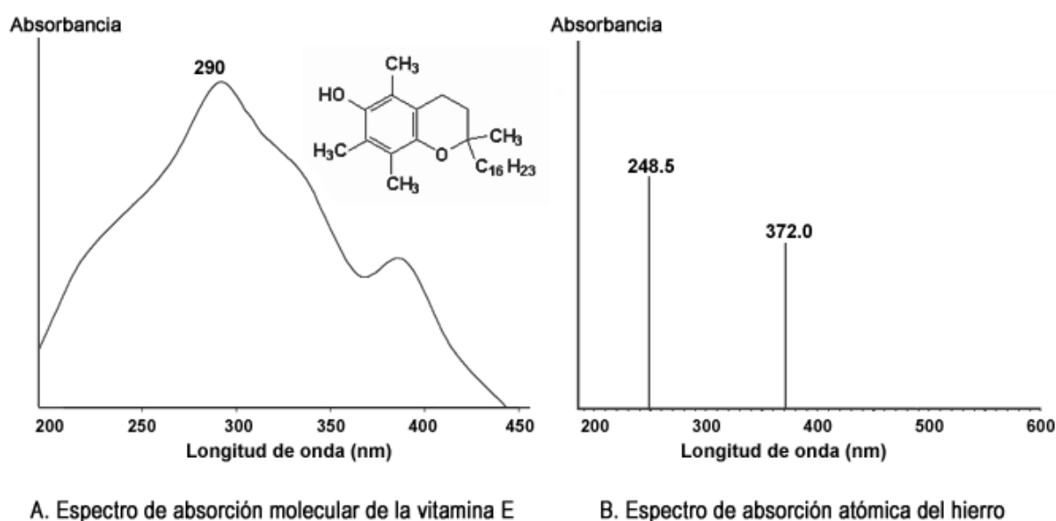
Figura 2.4. Espectros de absorción molecular y atómica en las regiones UV y visible.
