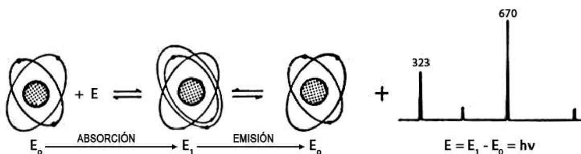
Figura 4.1. Procesos de absorción y emisión atómica.
