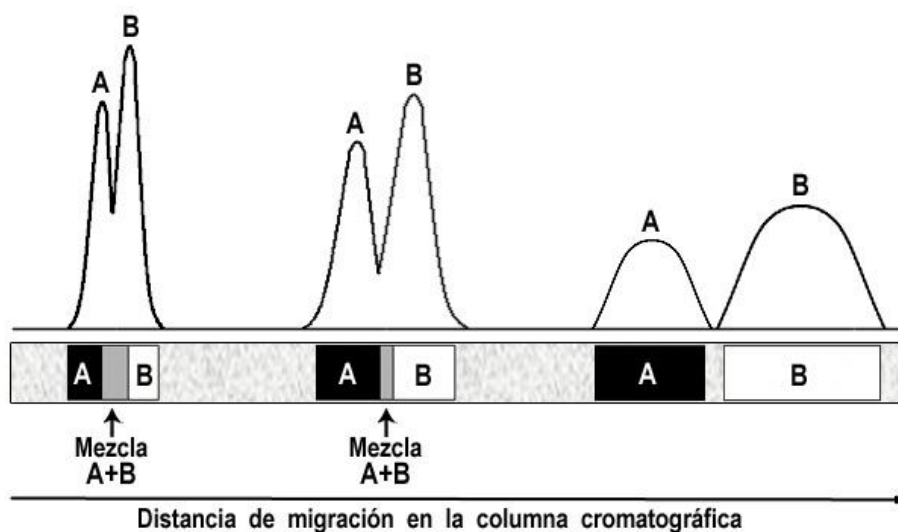
Figura 9.10. Proceso de migración de dos solutos (A y B) dentro de una columna cromatográfica
