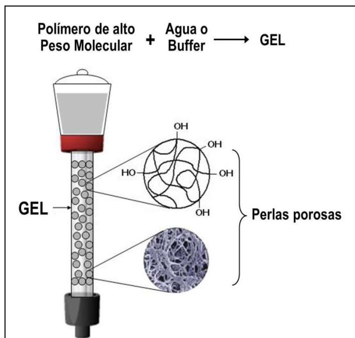
Figura 8.10. Estructura del gel para cromatografía de exclusión molecular
