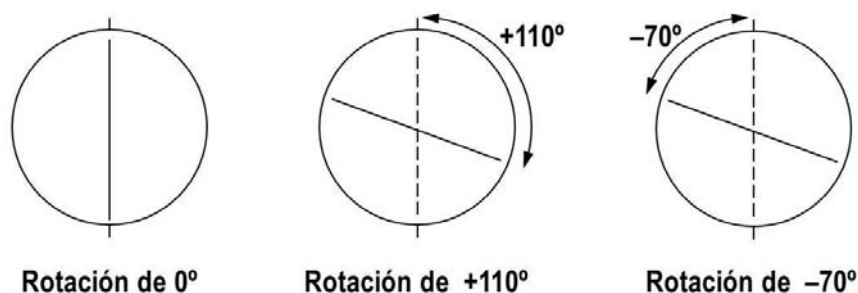
Figura 7.13. Ambigüedad del intervalo angular
