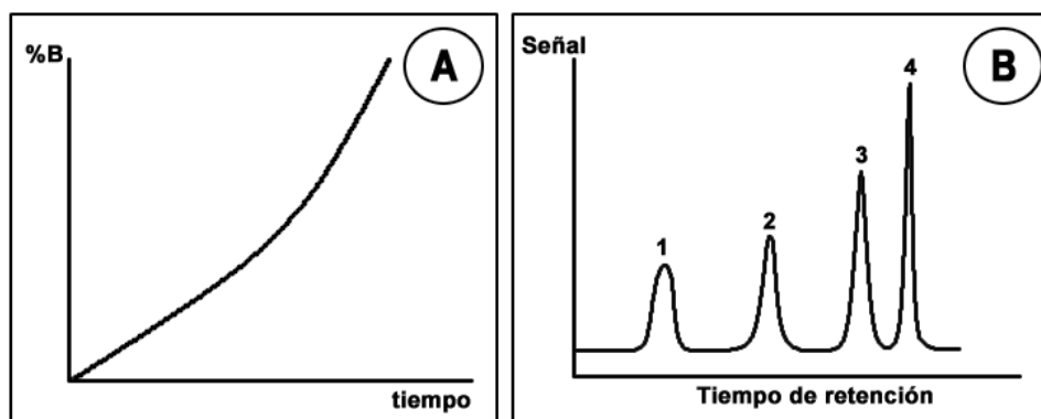
Figura 10.14. Gradiente exponencial: (A) representación gráfica, (B) cromatograma característico.
