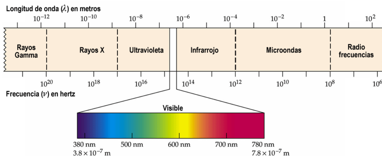
Figura 2.2. Regiones del espectro electromagnético.
