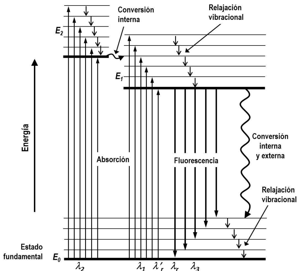
Figura 6.1. Diagrama de energía parcial para un sistema fluorescente
