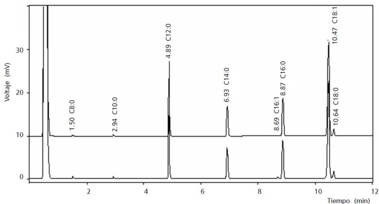
Figura 2. Superposición de perfiles cromatográficos de D-004 (superior) y D-004 sometido a condiciones de degradación (termólisis).
