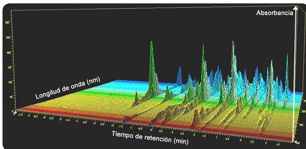
Figura 10.18. Gráfico tridimensional de una mezcla compleja obtenida con un detector de arreglo de diodos.
