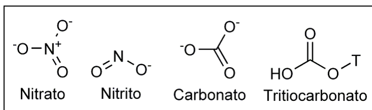
Figura 3.8. Especies absorbentes inorgánicas con transiciones n \rightarrow \pi^*
