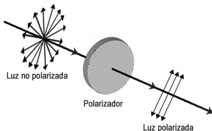
Figura 2.10. Una lámina polarizadora transforma la luz no polarizada en luz polarizada en un plano.
