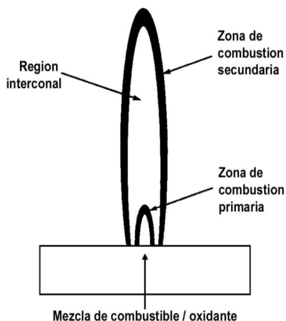
Figura 4.4. Regiones en una llama
