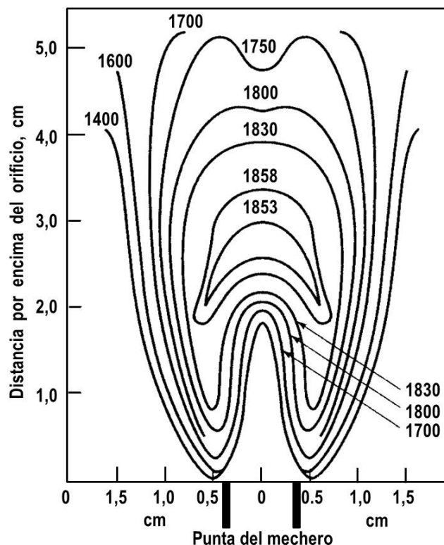
Figura 4.5. Perfiles de temperatura en °C en una llama de gas natural / aire
