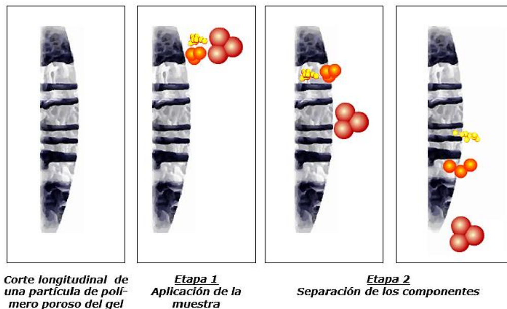
Figura 8.12. Mecanismo de exclusión molecular
