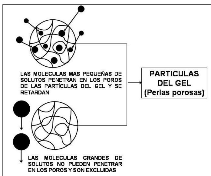
Figura 8.11. Proceso de exclusión molecular visto con aumento
