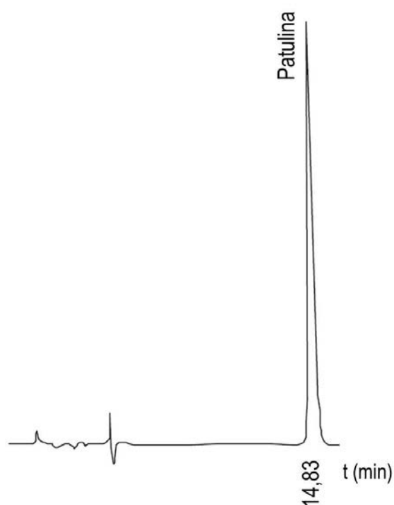
Figura 2. Cromatograma de un patrón de 24,8 ng de patulina.
