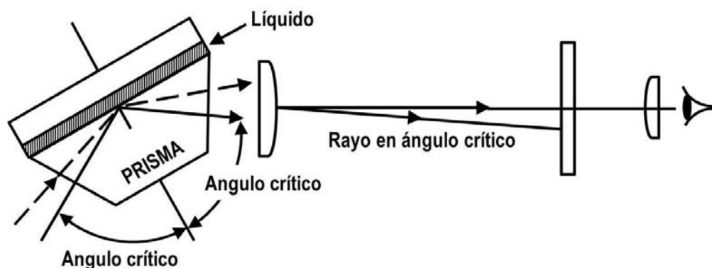
Figura 7.2. Representación esquemática del ángulo crítico
