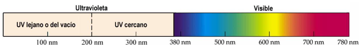
Figura 3.1. Regiones Ultravioleta y Visible del espectro electromagnético.
