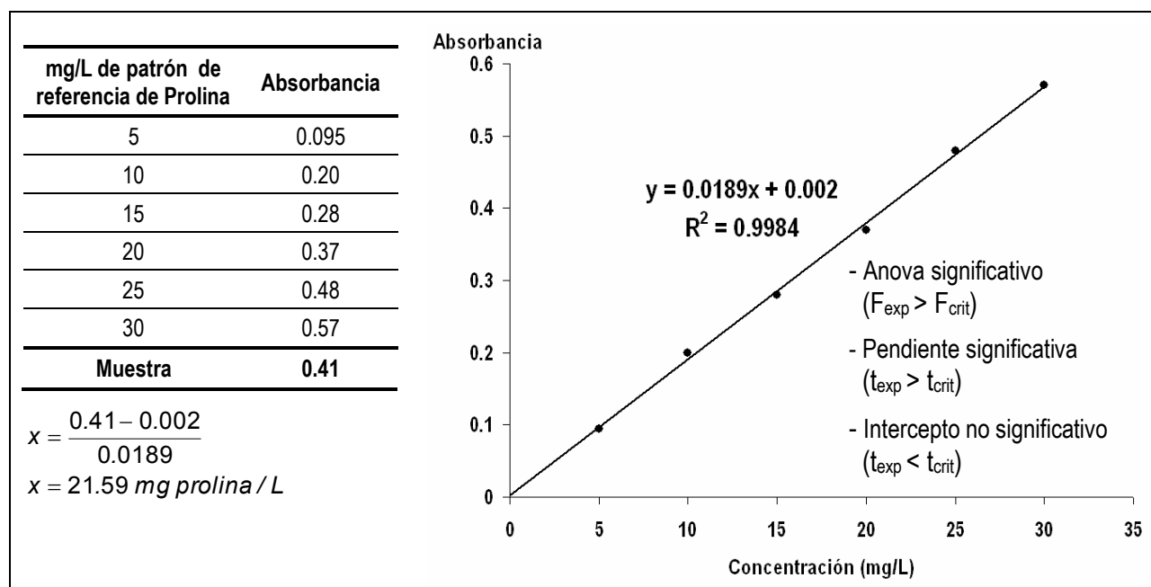
Figura 3.13b. Resultados obtenidos en el procesamiento de los datos experimentales de curva de calibración por el método de regresión lineal simple para la determinación de prolina en jugo de uvas.
