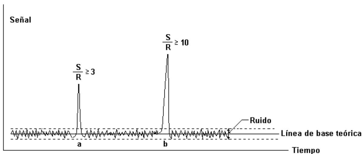
Figura 10.23. Criterios para la determinación del LD (a) y el LC
