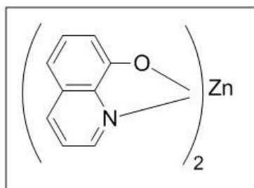
Figura 6.4. Complejo de la 8-hidroxiquinolina con el Cinc.
