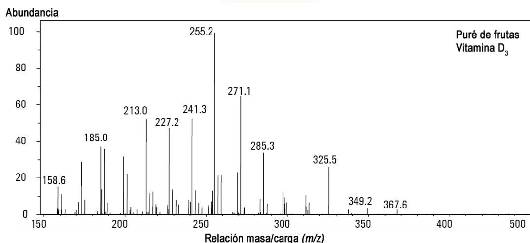
Figura 10.8. Espectro de masa obtenido para la Vitamina D 3 (colecalfiferol)
