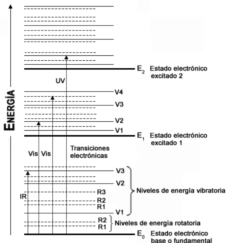
Figura 2.5. Diagrama parcial de los niveles energéticos para una molécula.
