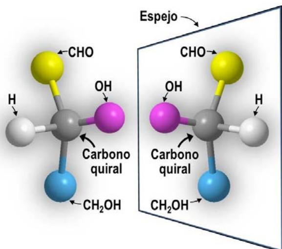
Figura 7.10. Estructura simplificada del D (+) gliceraldehído (a la izquierda de la figura) y su imagen especular no superponible, el L (-) gliceraldehído (a la derecha).
