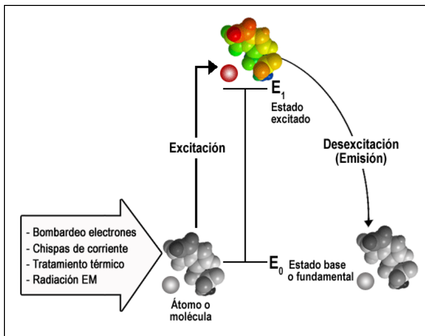
Figura 2.6. Representación esquemática del proceso de emisión de radiación
