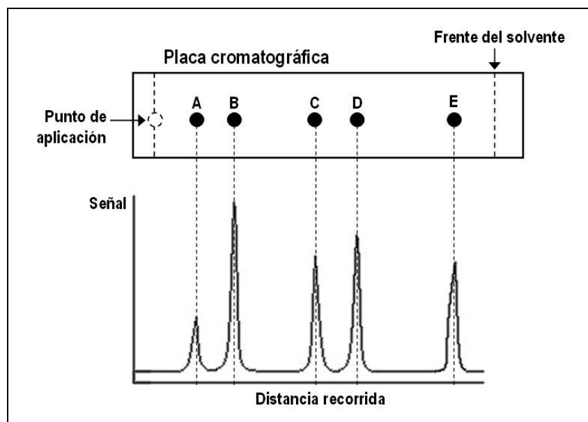
Figura 12.18. Placa cromatográfica de una muestra de cinco componentes (A, B, C, D y E) y cromatograma obtenido por barrido densitométrico.
