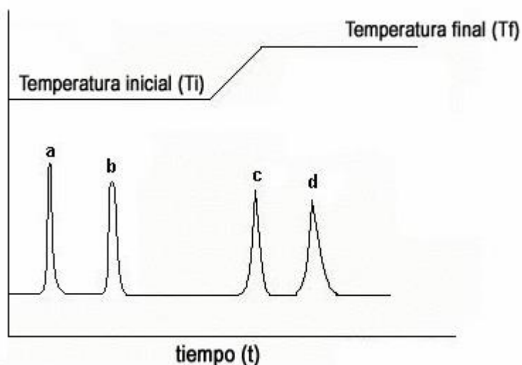
Figura 11.9. Cambio en el valor de la temperatura de operación. S= señal del solvente
