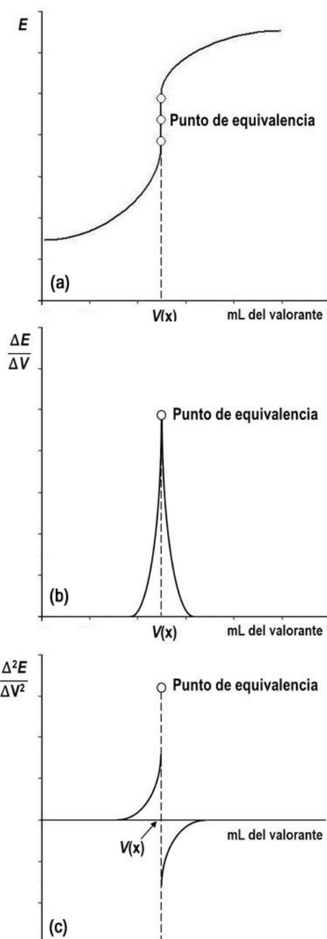
Figura 13.8. Curvas de valoración potenciométrica
