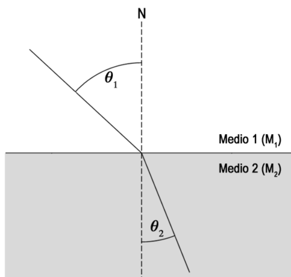
Figura 2.8. Refracción de la luz al pasar del medio M_1 menos denso al medio M_2 más denso en el cual su velocidad es menor
