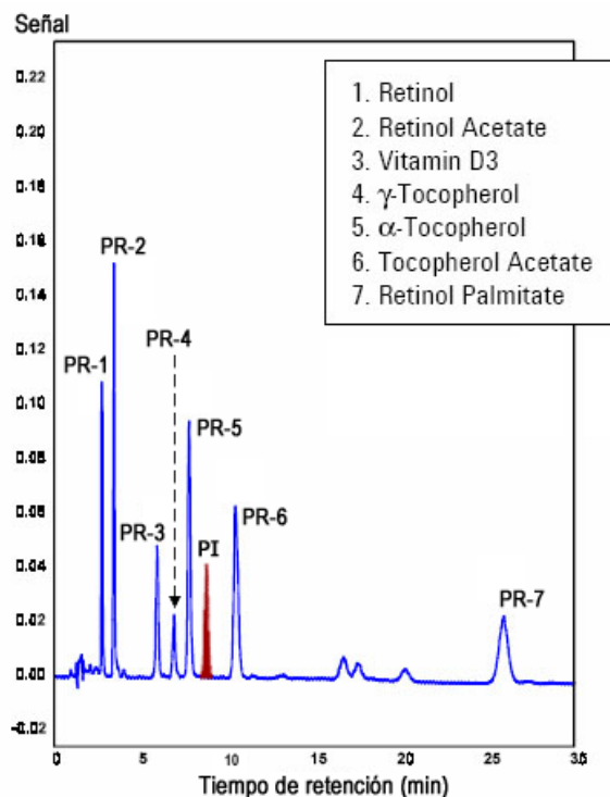
Figura 10.22. Cromatograma de la mezcla de los 7 patrones de referencia de las vitaminas (PR) y el patrón interno (PI)
