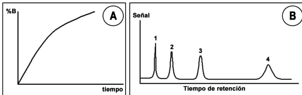
Figura 10.13. Gradiente logarítmico: (A) representación gráfica, (B) cromatograma característico.
