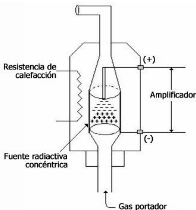
Figura 11.15. Detector de captura electrónica (ECD)
