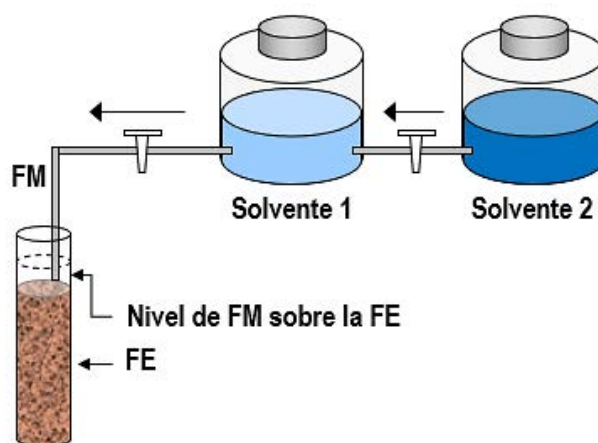
Figura 9.3. Gradiente de polaridad ascendente
