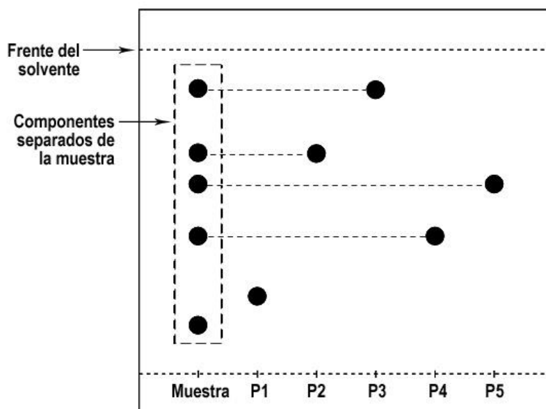
Figura 12.4. Cromatograma revelado de una muestra de 5 componentes. Nótese que 4 de ellos han podido ser identificados, correspondiéndose con los patrones P2, P3, P4 y P5. Véase además que el componente de la muestra de mayor afinidad con la fase estacionaria (que mostró el menor recorrido) no pudo ser identificado en esta corrida puesto que su distancia de recorrido no coincide con la de ninguno de los patrones aplicados. Así mismo el patrón P1 no está presente en la muestra.
