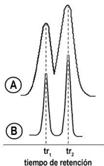
Figura 9.12. Efecto del ensanchamiento de banda sobre la resolución
