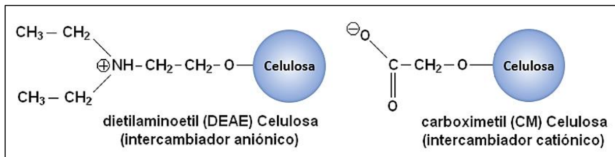
Figura 8.9. Estructura de dos resinas intercambiadoras en soporte de celulosa
