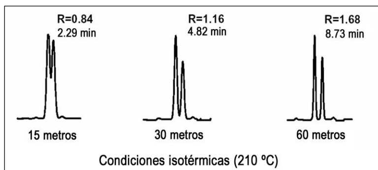
Figura 11.5. Efecto de la longitud de la columna sobre la resolución.
