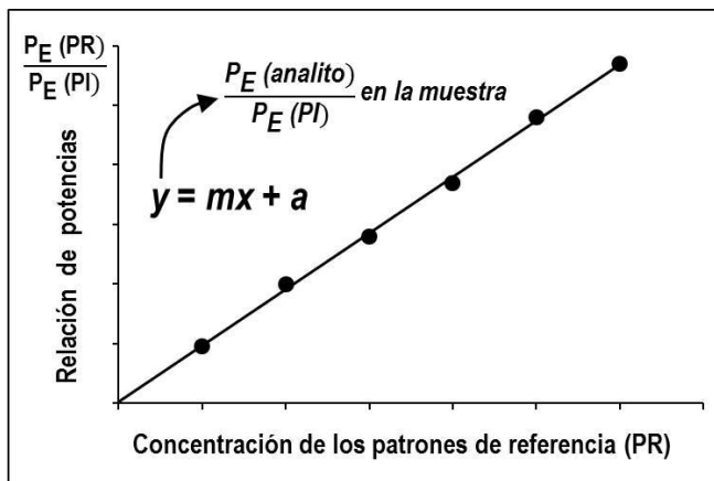
Figura 5.6. Gráfico de calibración por el método del patrón interno. P_E (PR) es la potencia emitida de los patrones de referencia y P_E (PI) es la potencia emitida del patrón interno.
