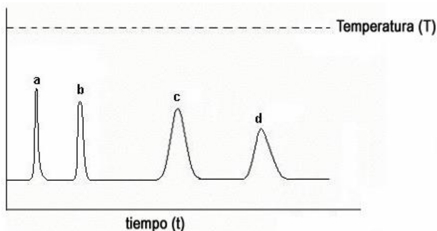
Figura 11.8. Cromatograma isotérmico de una mezcla con diferencias grandes en los puntos de ebullición de los componentes separados.
