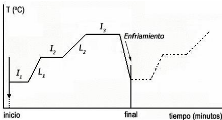
Figura 11.11. Programa complejo de ciclo de programación o rampas de temperaturas. I_1 representa una operación isotérmica inicial. L_1 muestra un ascenso lineal de la temperatura, E representa la etapa de enfriamiento. En la mayoría de los equipos puede prefijarse las temperaturas y duraciones de I_1 , I_2 , I_3 , etc. Así como las velocidades de ascenso de la temperatura en las etapas L_1 , L_2 , etc., dentro de rangos bastantes amplios.
