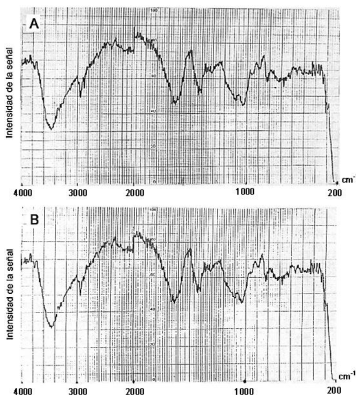
Figura 2. Espectros IR del alginato cubano (A) y del alginato mexicano (B).
