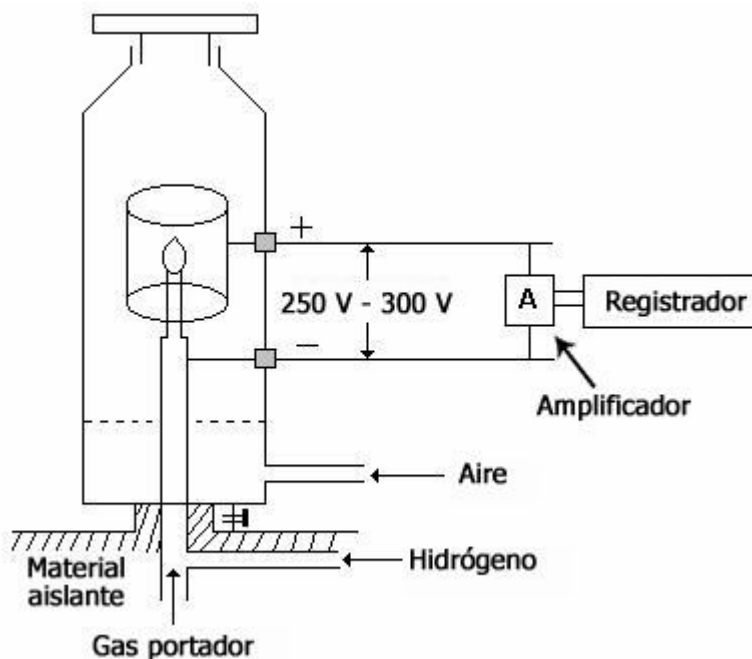
Figura 11.14. Detector de ionización por llama (FID)
