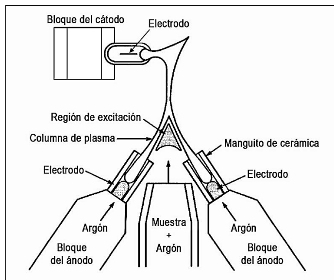
Figura 5.5. Fuente de plasma de corriente continua de tres electrodos
